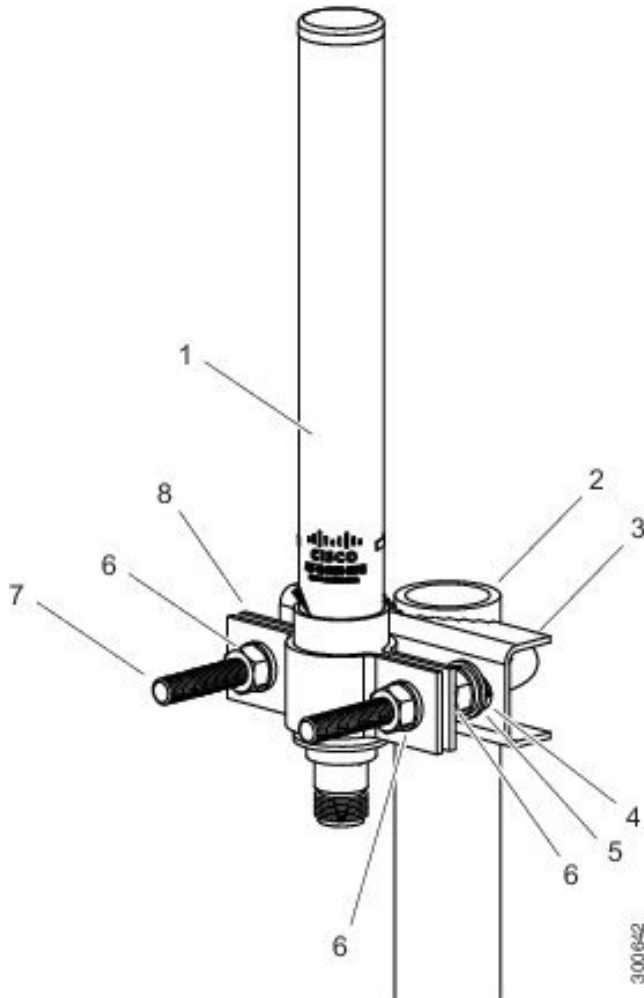
図 2: アンテナ詳細
