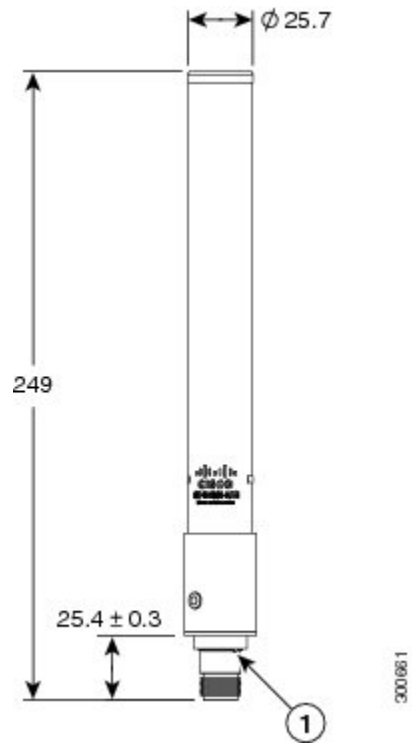
図 1: 屋外用無指向性アンテナ
