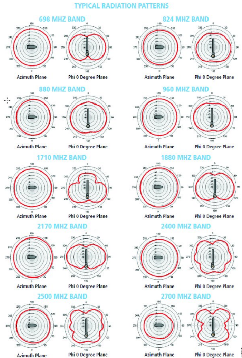
図 2: 関節付きダイポールアンテナの放射パターン
