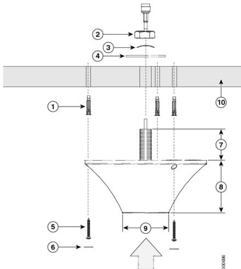
図 3: アンテナ詳細
