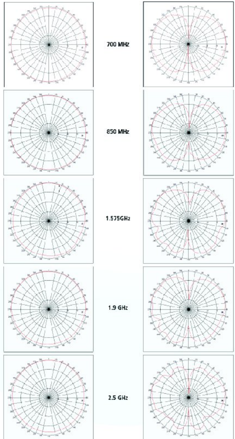
図 2: 4G Volcano アンテナ放射パターン
