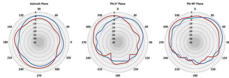
図 7: 1710 MHz セルラーアンテナ放射パターン
