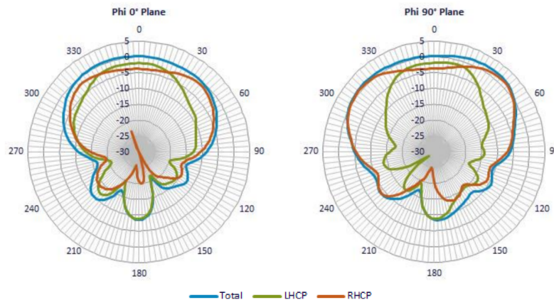
図 10: 1575 MHz GPS アンテナ放射パターン
