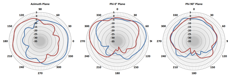
図 10: 1575 MHz GPS アンテナ放射パターン
