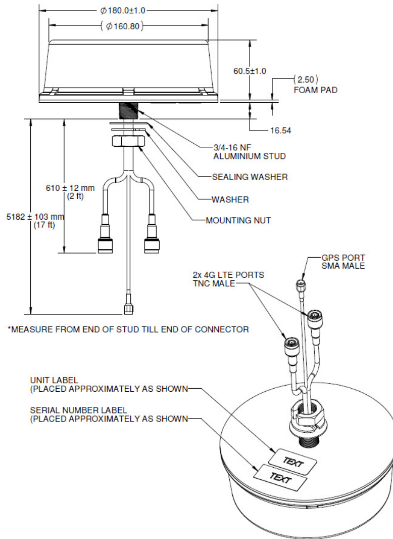
図 2: Cisco ANT-3-4G2G1-0 の機械的詳細
