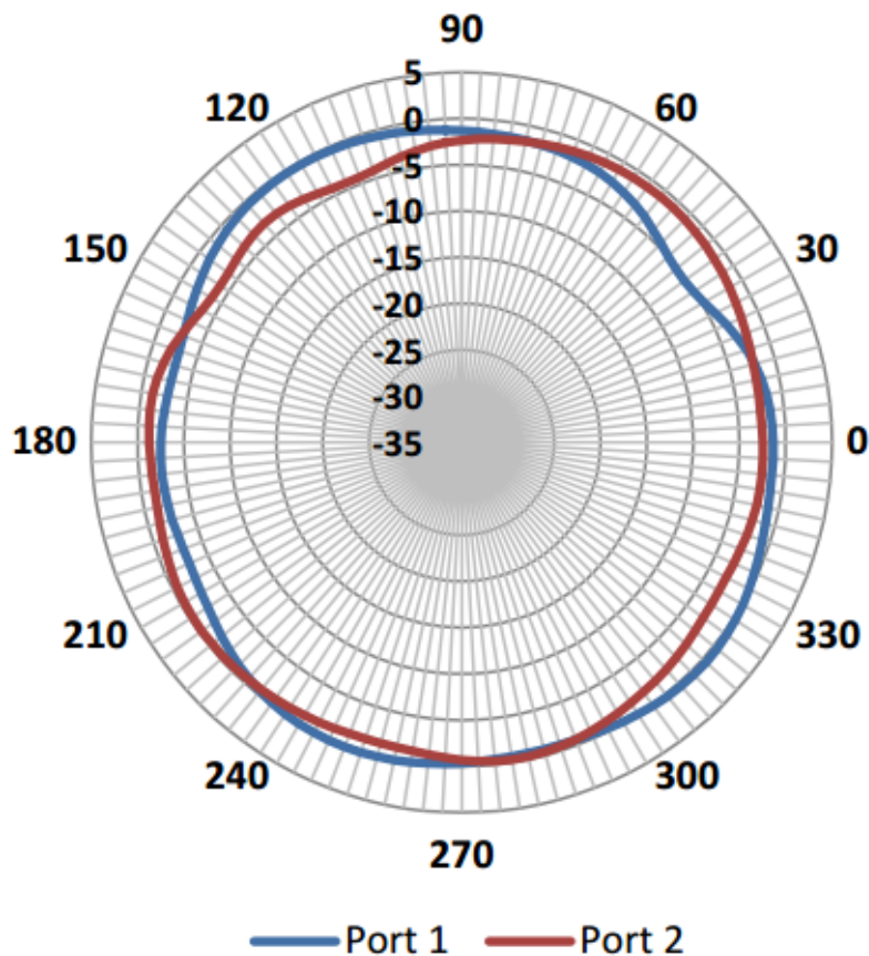
図 4: 2.46 GHz アンテナ放射パターン - 垂直面
