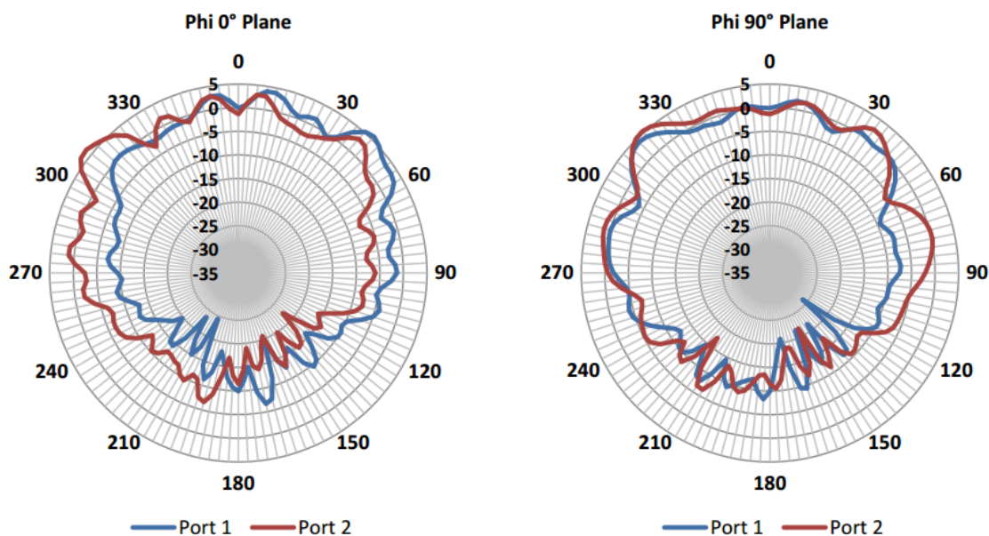
図 8: 5.55 GHz アンテナ放射パターン - 垂直面
