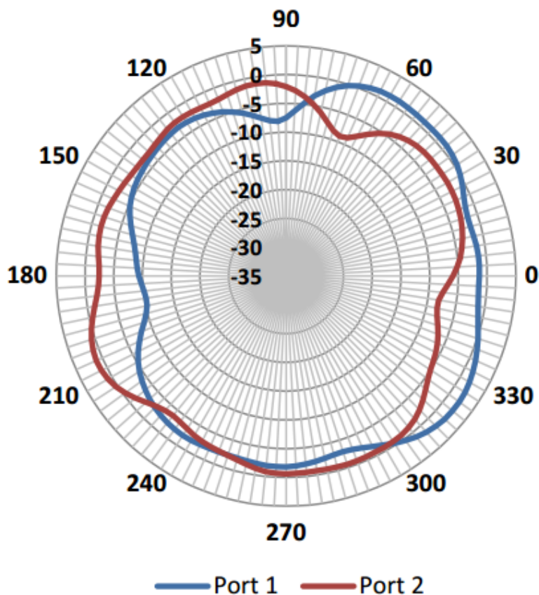
図 8: 5.55 GHz アンテナ放射パターン - 垂直面
