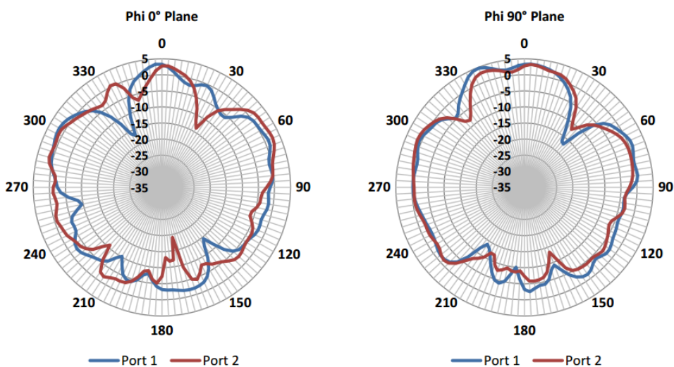
図 4: 2.46 GHz アンテナ放射パターン - 垂直面
