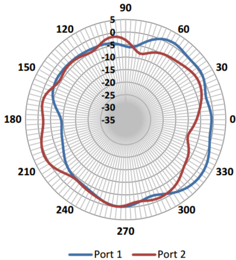
図 10: 5.9 GHz アンテナ放射パターン - 垂直面
