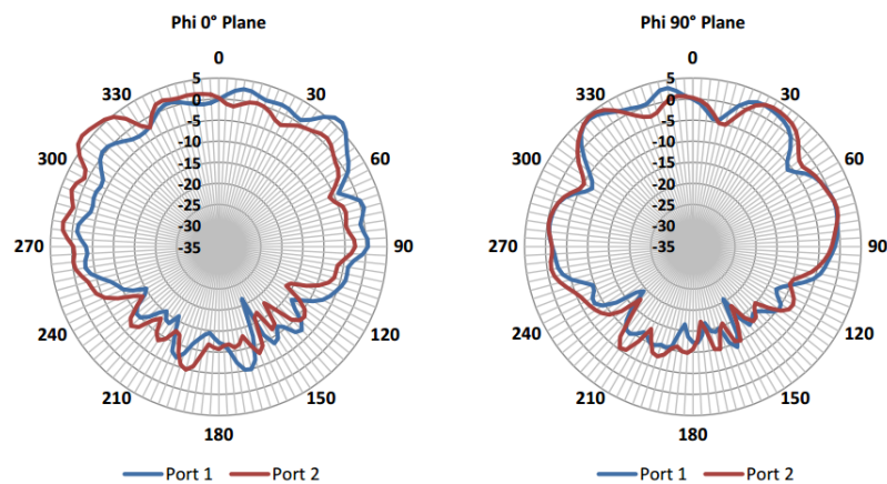
図 6: 4.9 GHz アンテナ放射パターン - 垂直面
