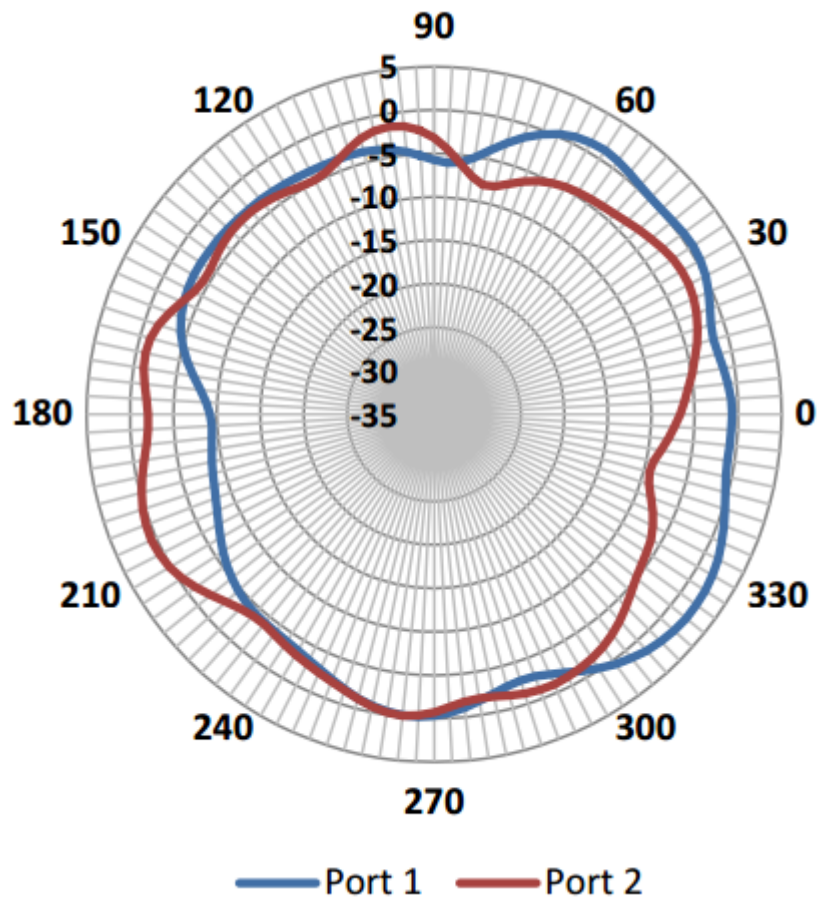
図 6: 4.9 GHz アンテナ放射パターン - 垂直面
