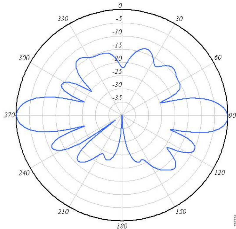
図 2: 仰角面内放射パターン
