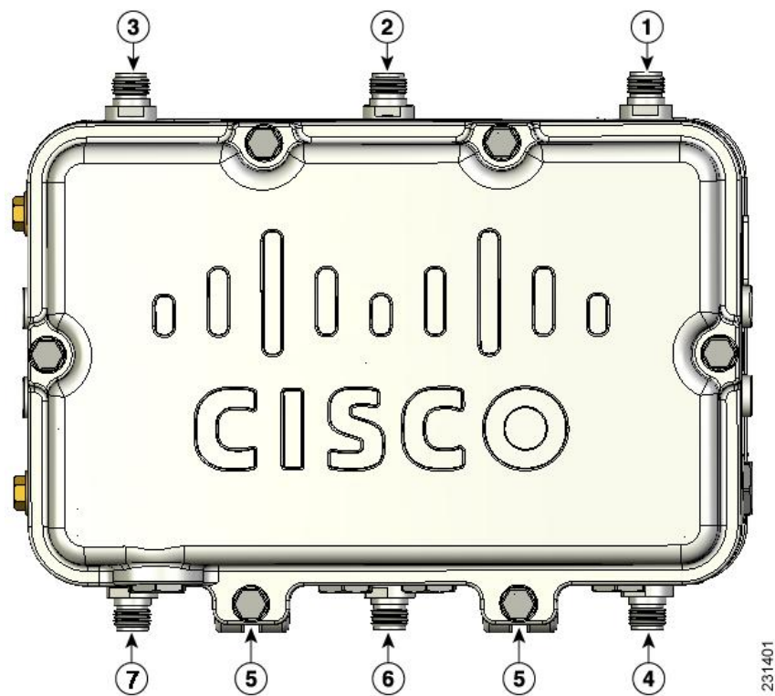
図 5: アンテナ ポートの位置
