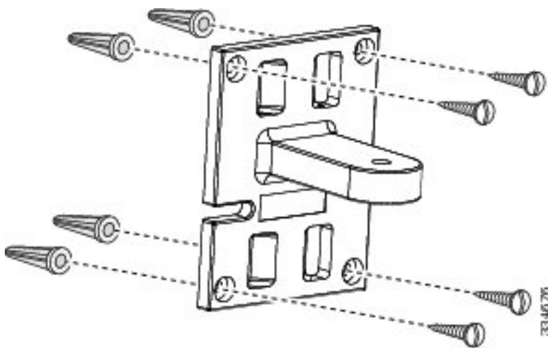
図 10: 壁面への取り付け
