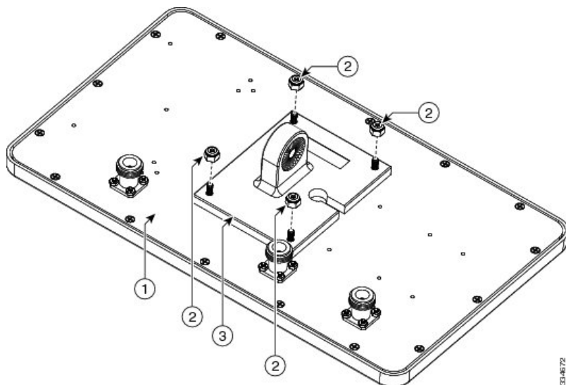
図 6: アンテナ マウント ブラケットの取り付け
