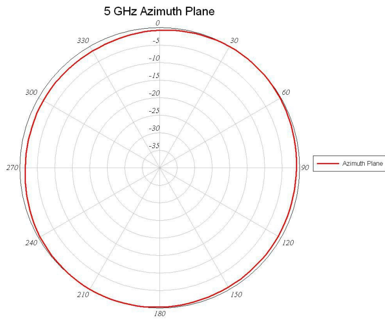
図 3: 方位角面内放射パターン (5 GHz)
