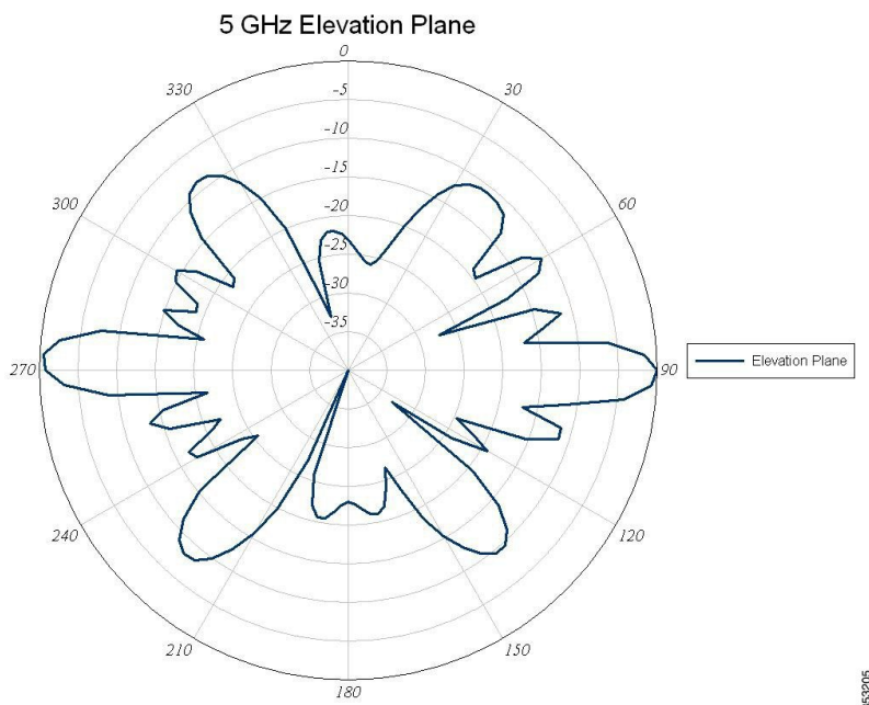
図 4: 仰角面内放射パターン (5 GHz)
