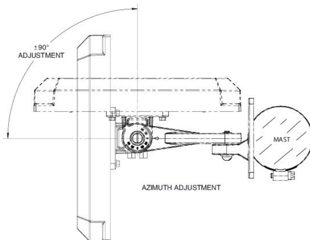
図 6: 方位角調整
