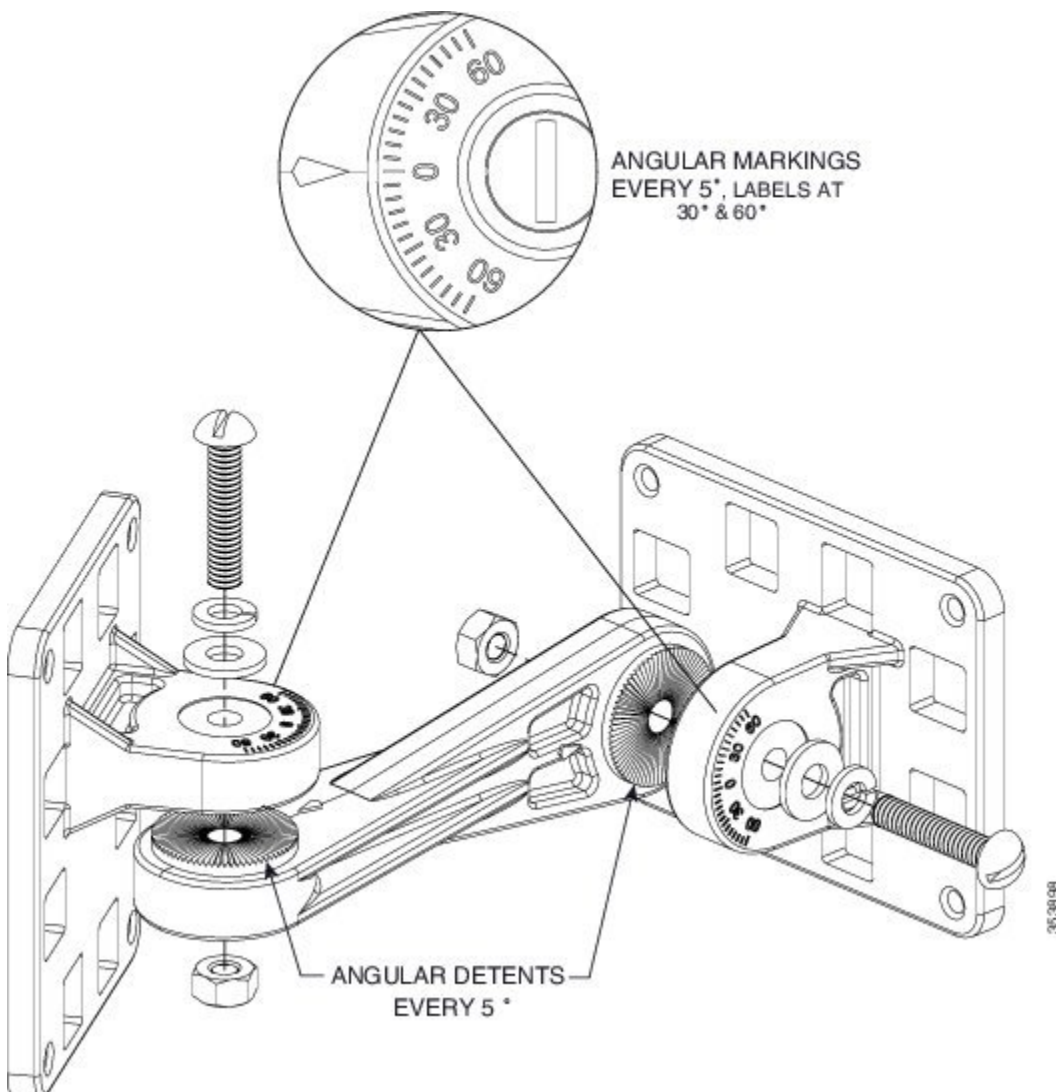
図 8: 方位角調整ピボットおよび仰角調整ピボットの拡大図
