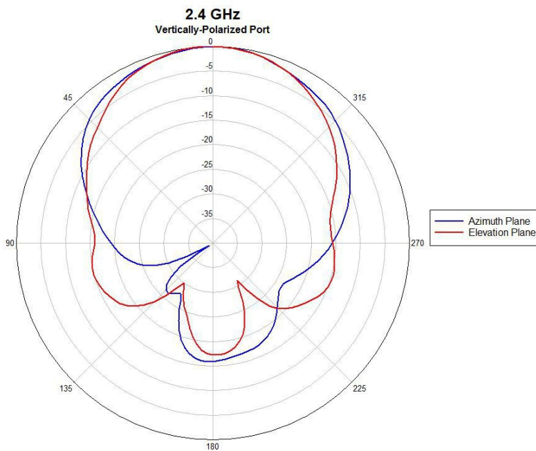
図 2: 2.4 GHz 垂直
