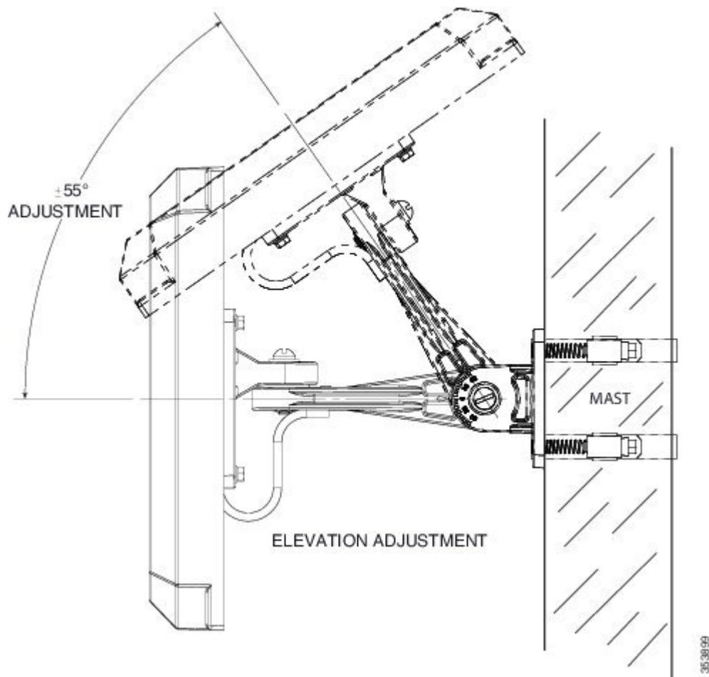
図 7: 仰角調整
