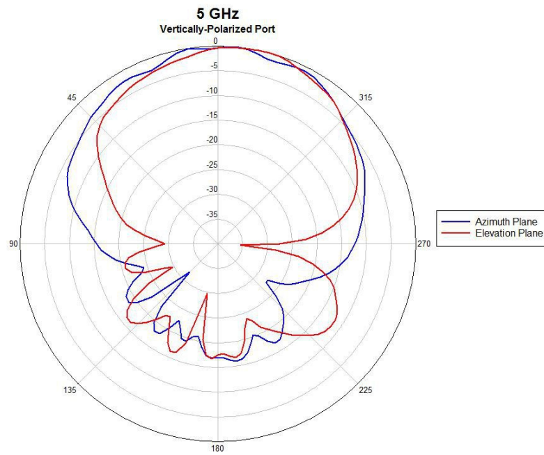
図 4: 5 GHz 垂直
