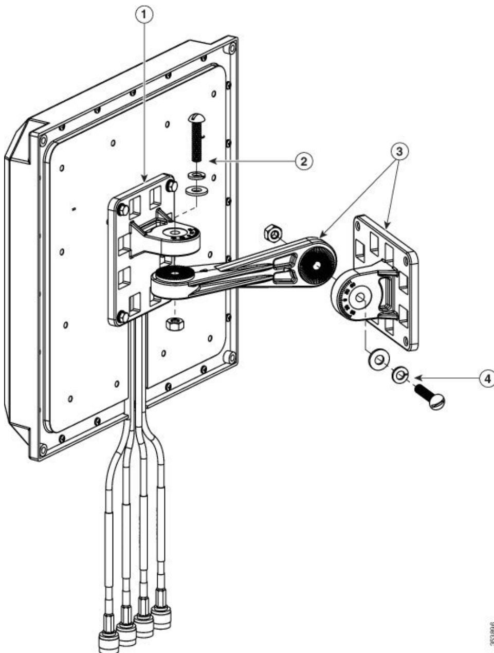
図 5: アンテナおよびブラケット金具のアセンブリの分解図
