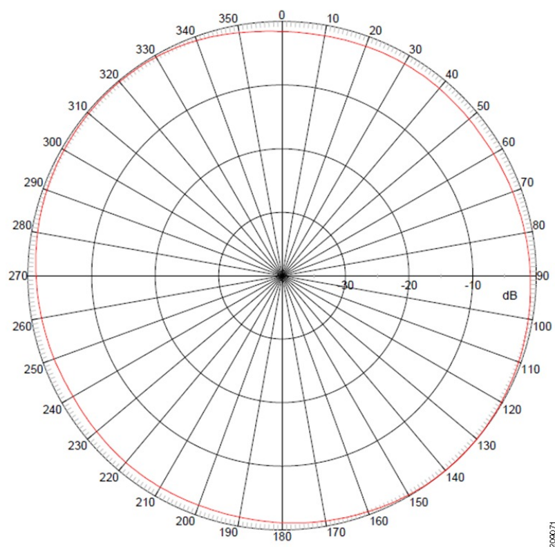
図 1: 方位角面内放射パターン (2.4 GHz)
