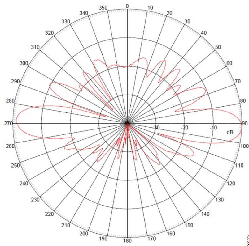
図 4: 仰角面内放射パターン (5 GHz)
