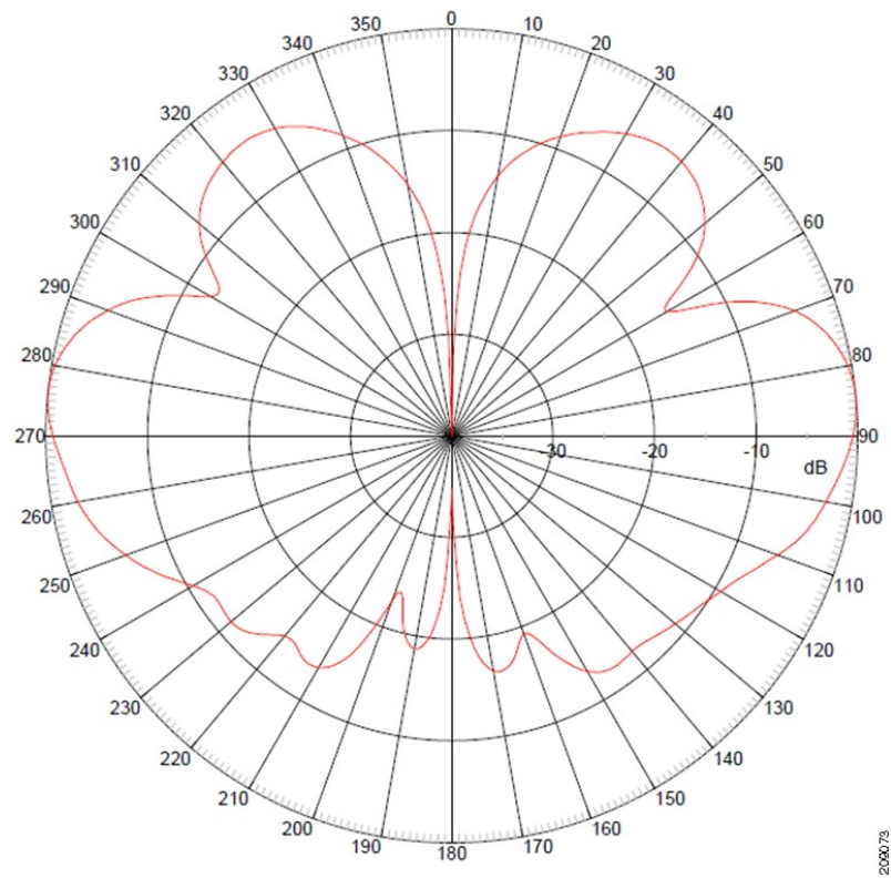
図 2: 仰角面内放射パターン (2.4 GHz)
