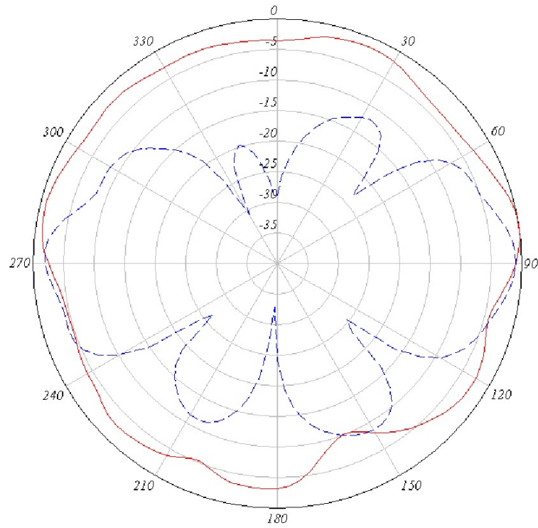
図 6: 5 GHz アンテナ 3 の方位角面および仰角面パターン
