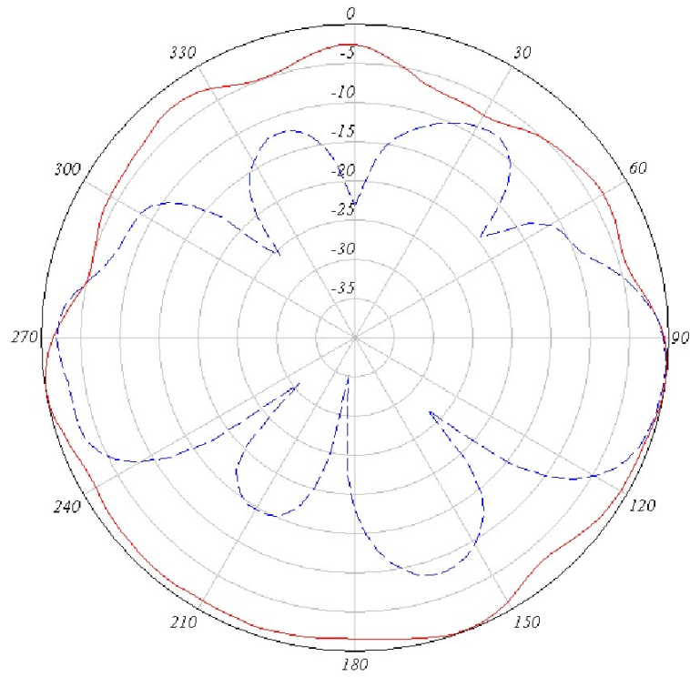
図 4: 5 GHz アンテナ 2 の方位角面および仰角面パターン
