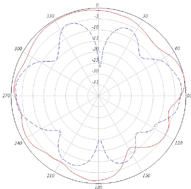
図 8: 5 GHz アンテナ 4 の方位角面および仰角面パターン
