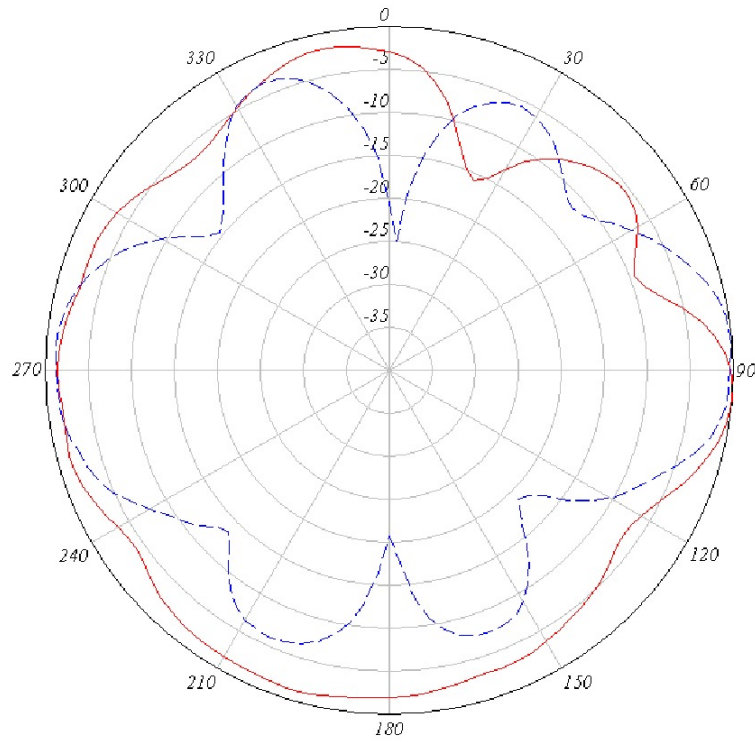
図 2: 5 GHz アンテナ 1 の方位角面および仰角面パターン
