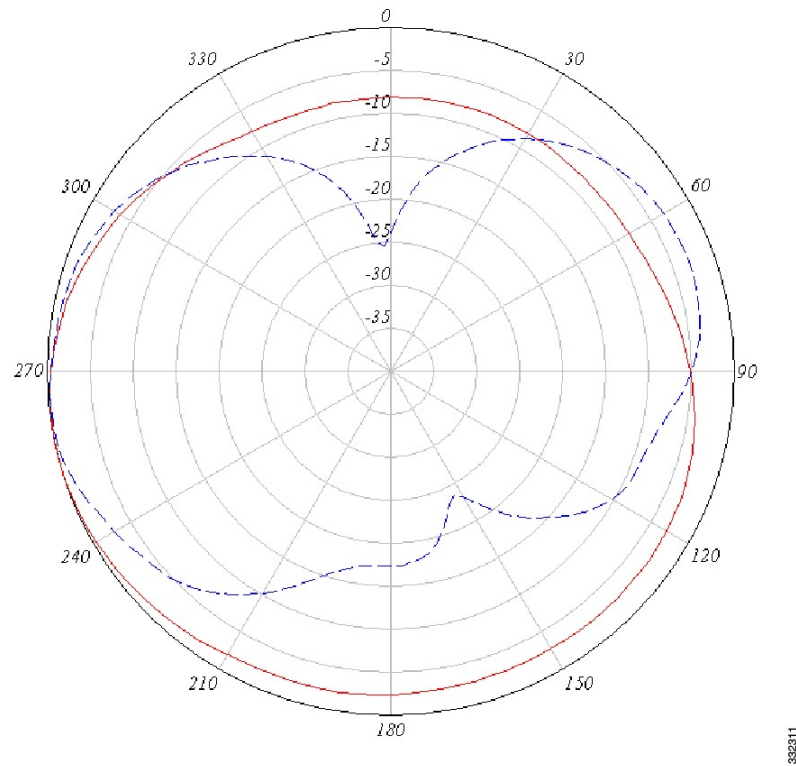
図 1: 2.4 GHz アンテナ 1 の方位角面および仰角面パターン
