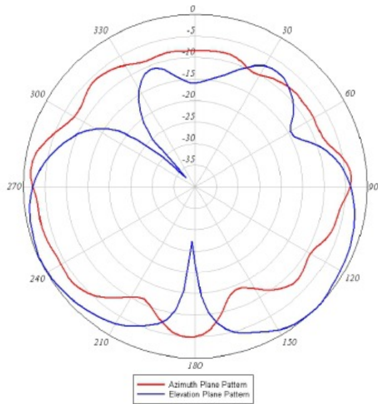
図 4: 5 GHz 素子 2 の方位角面および仰角面パターン
