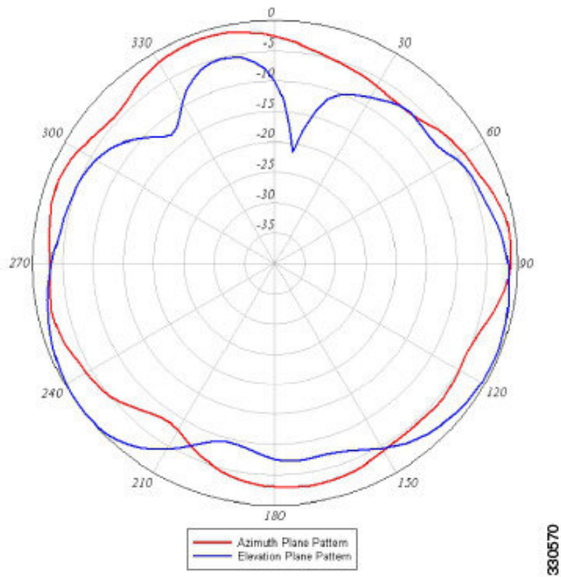
図 7: 2.4 GHz 素子 4 の方位角面および仰角面パターン
