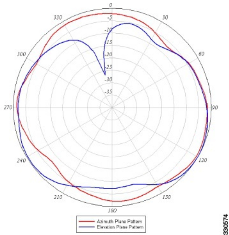
図 3: 2.4 GHz 素子 2 の方位角面および仰角面パターン
