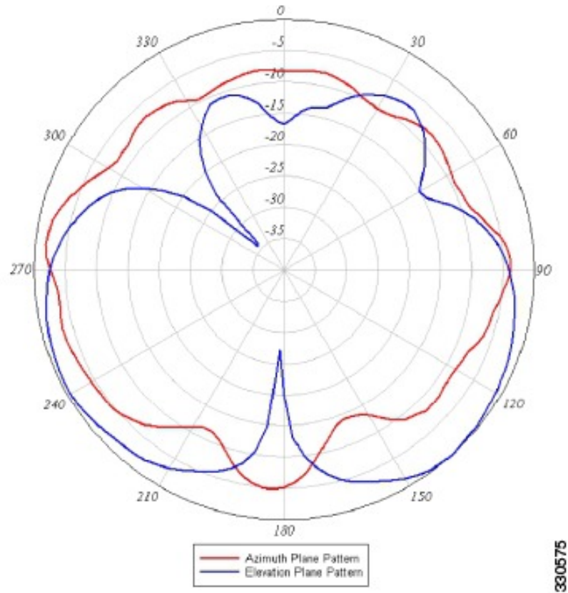
図 2: 5 GHz 素子 1 の方位角面および仰角面パターン
