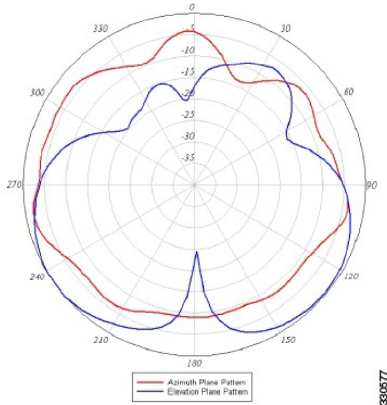
図 8: 5 GHz 素子 4 の方位角面および仰角面パターン
