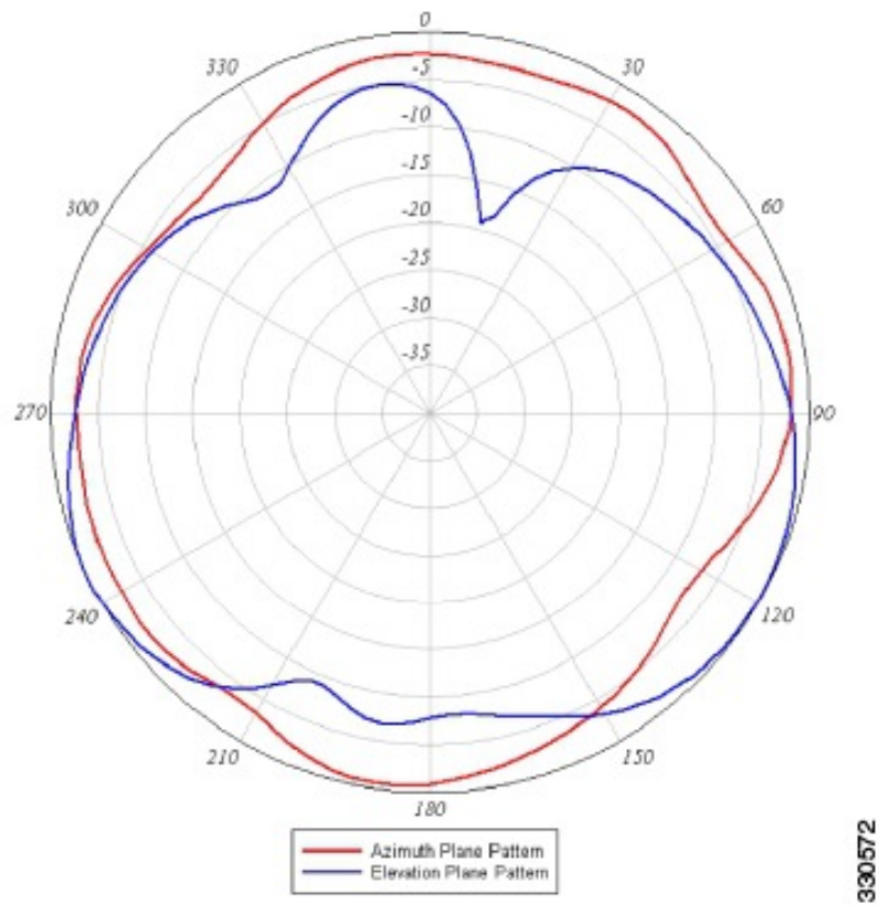
図 5: 2.4 GHz 素子 3 の方位角面および仰角面パターン
