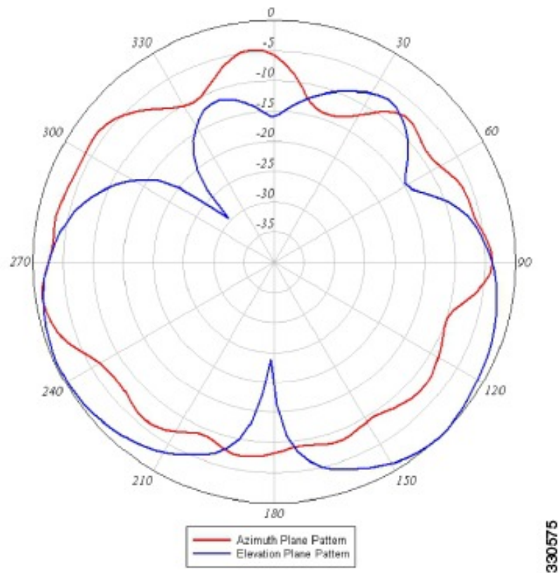
図 6: 5 GHz 素子 3 の方位角面および仰角面パターン
