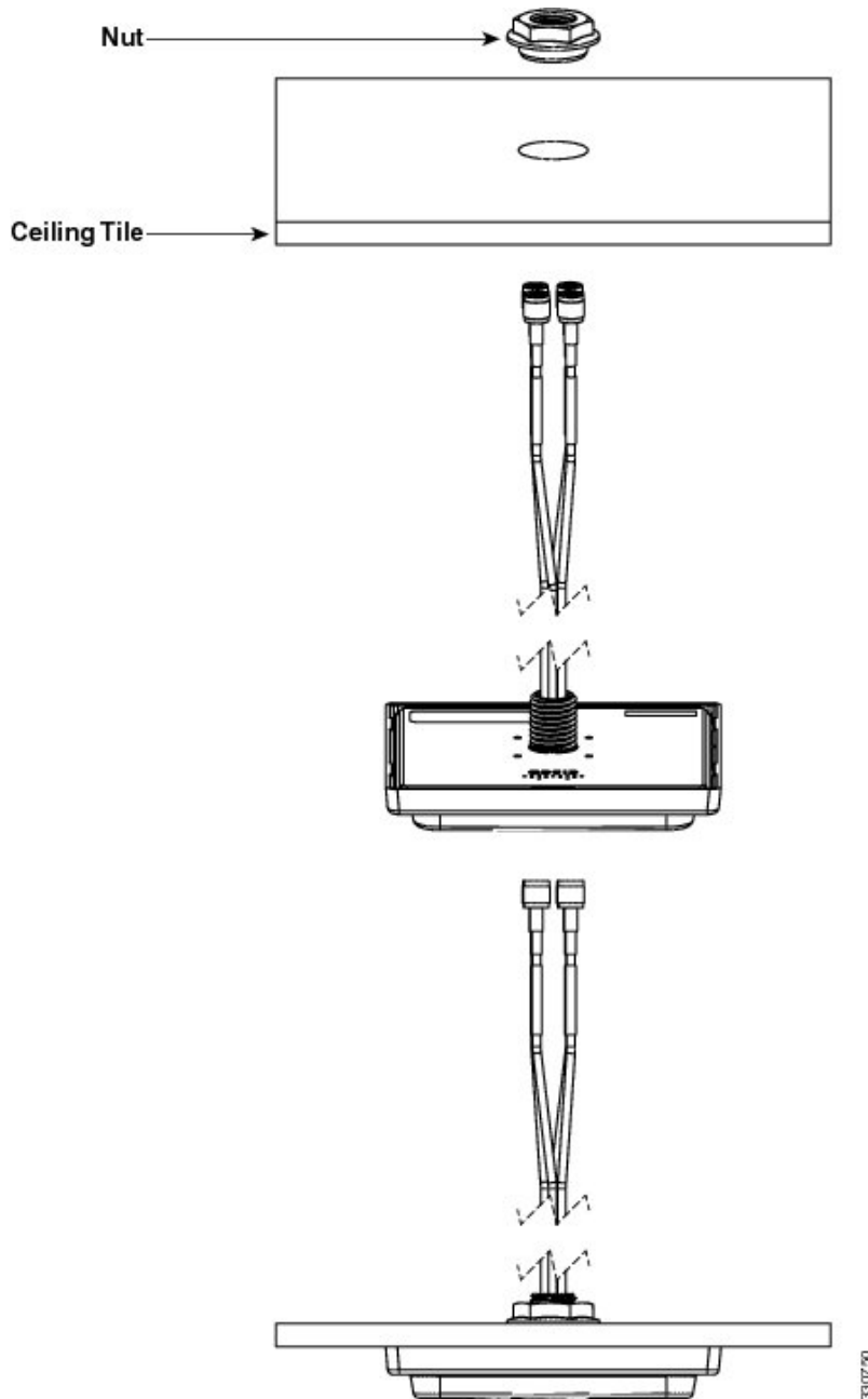
図 9: 天井タイルへの取り付けの詳細
