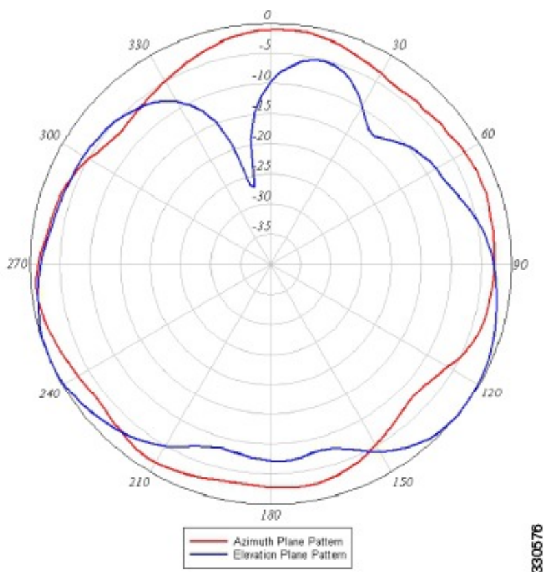
図 1: 2.4 GHz 素子 1 の方位角面および仰角面パターン
