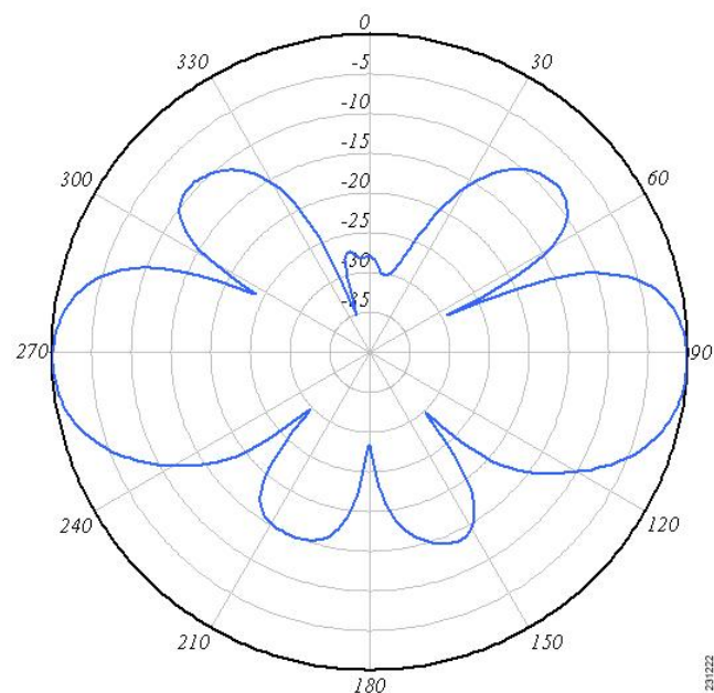
図 2: 仰角面内放射パターン
