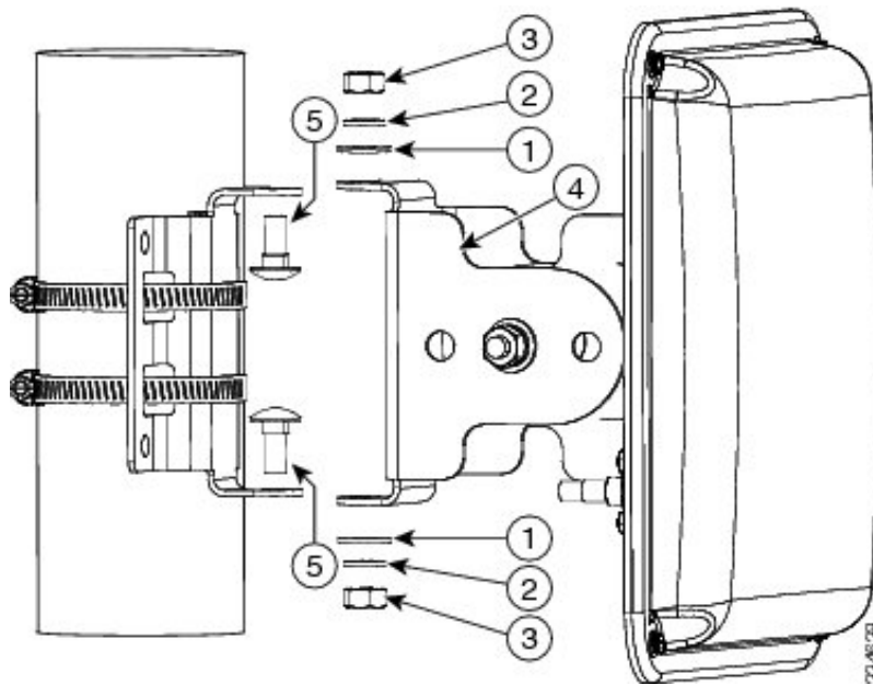
図 11: アンテナ アセンブリの取り付け
