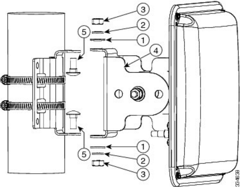
図 5: アンテナ アセンブリの取り付け
