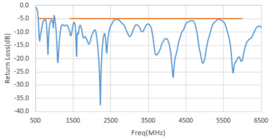
反射損失（曲げ時）
