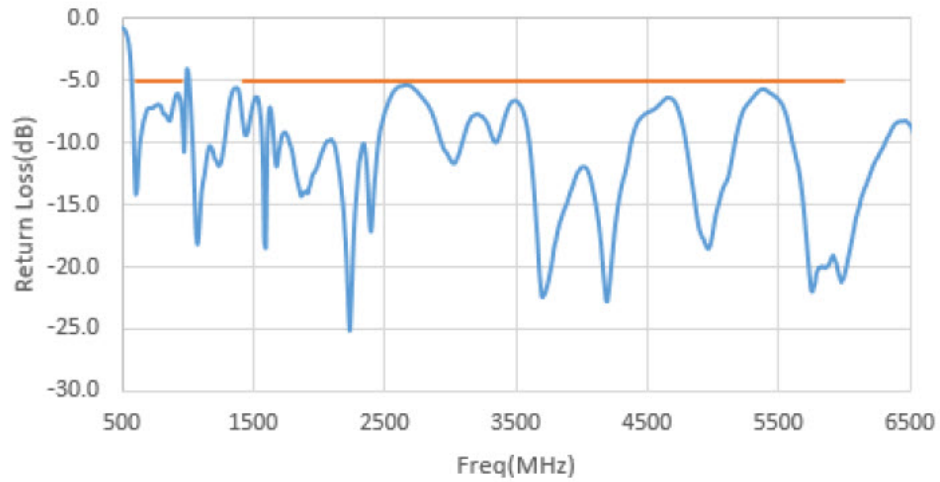
反射損失（曲げ時）
