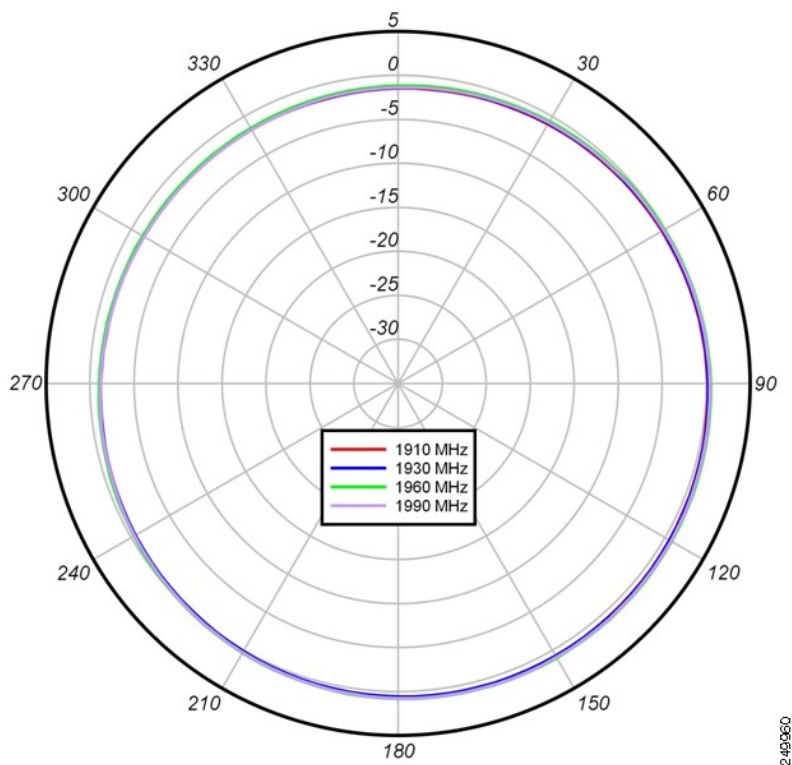
図 9: 1900 MHz 帯域での方位角面パターン
