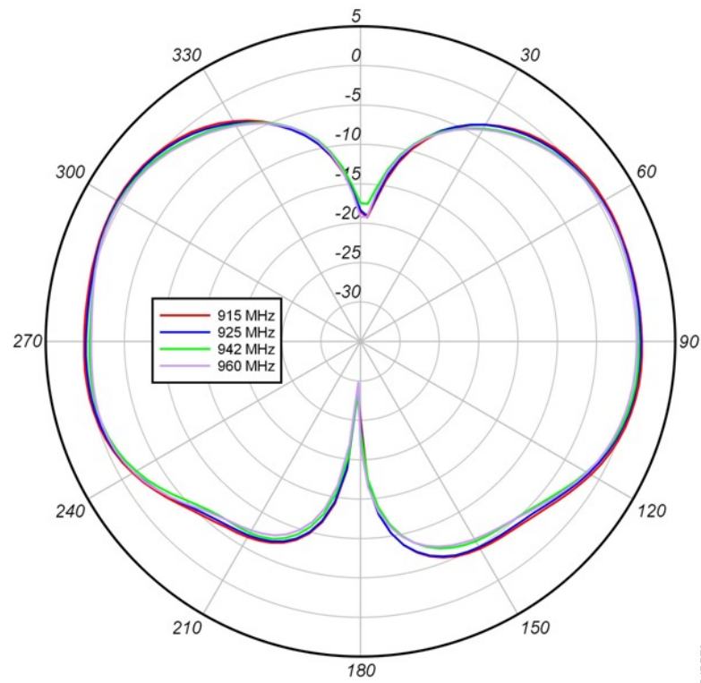
図 22: 900 MHz 帯域での仰角面パターン ( \Phi = 90 度断面)
