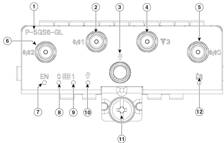
図 3: 5G プラガブルインターフェイス モジュール - P-5GS6-GL
