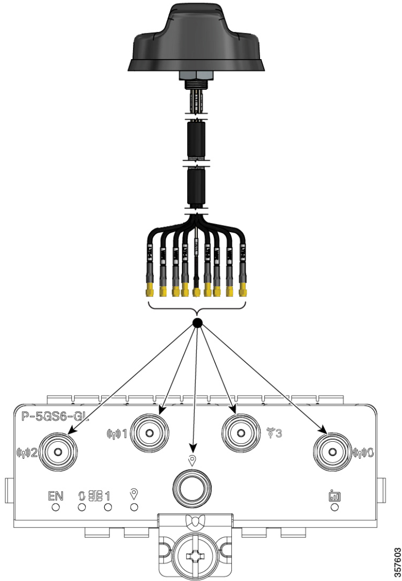
図 5: 5G NR アンテナ (5G-ANTM-04-B) を P-5GS6-GL PIM に取り付ける
