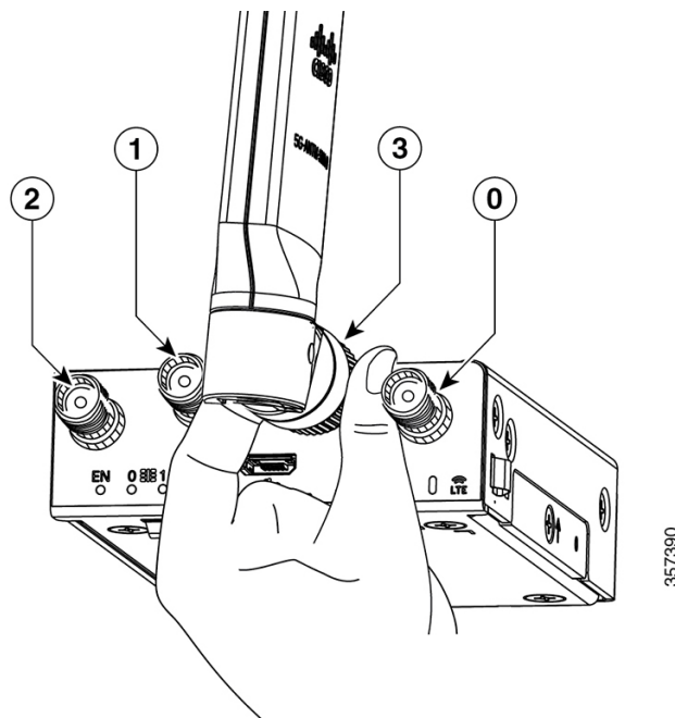
図 4: アンテナの取り付け
