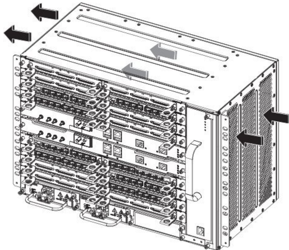
図 1: Cisco ASR 907 ルータのシャーシのエアー フロー
