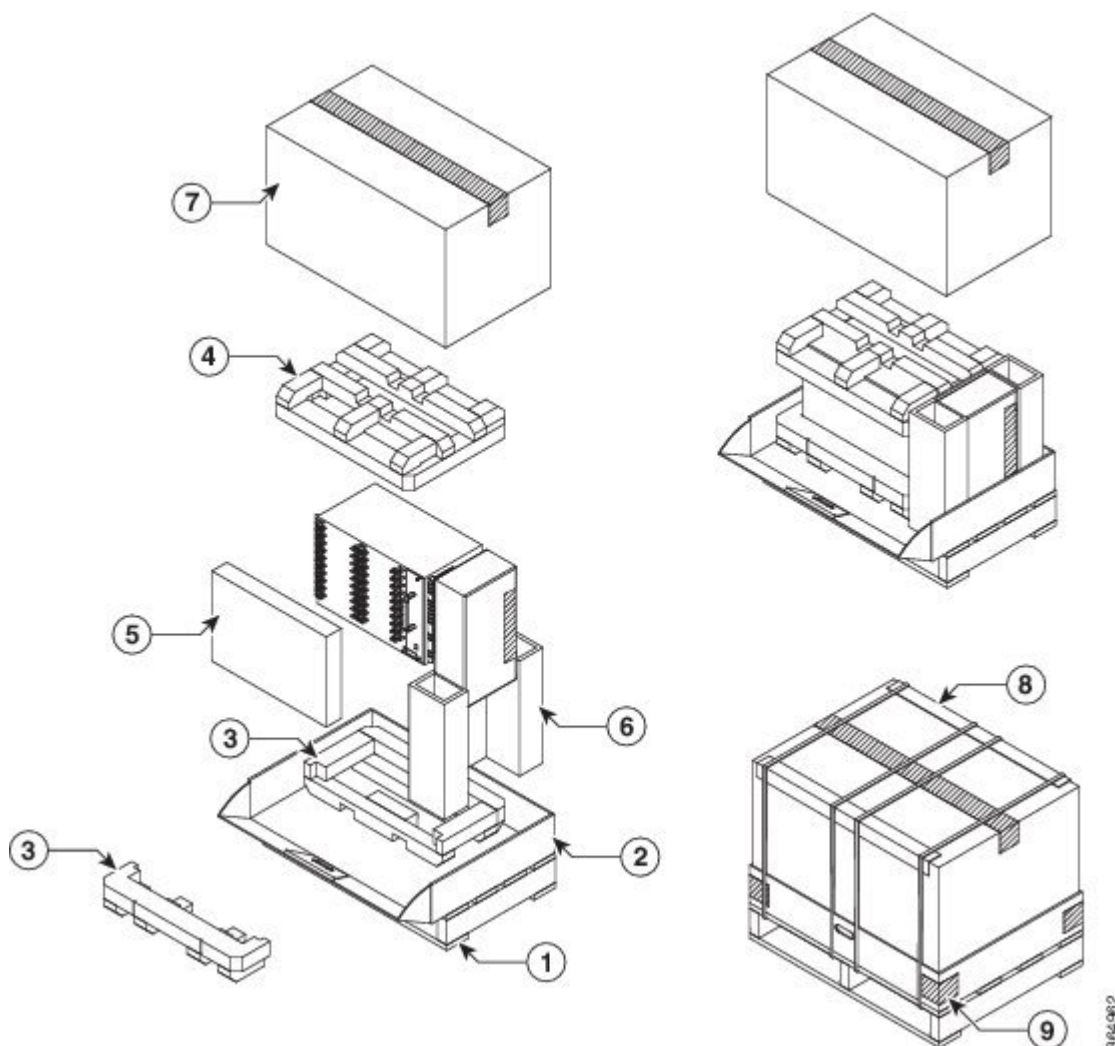
図 4: Cisco ASR 907 ルータの輸送用パッケージ
