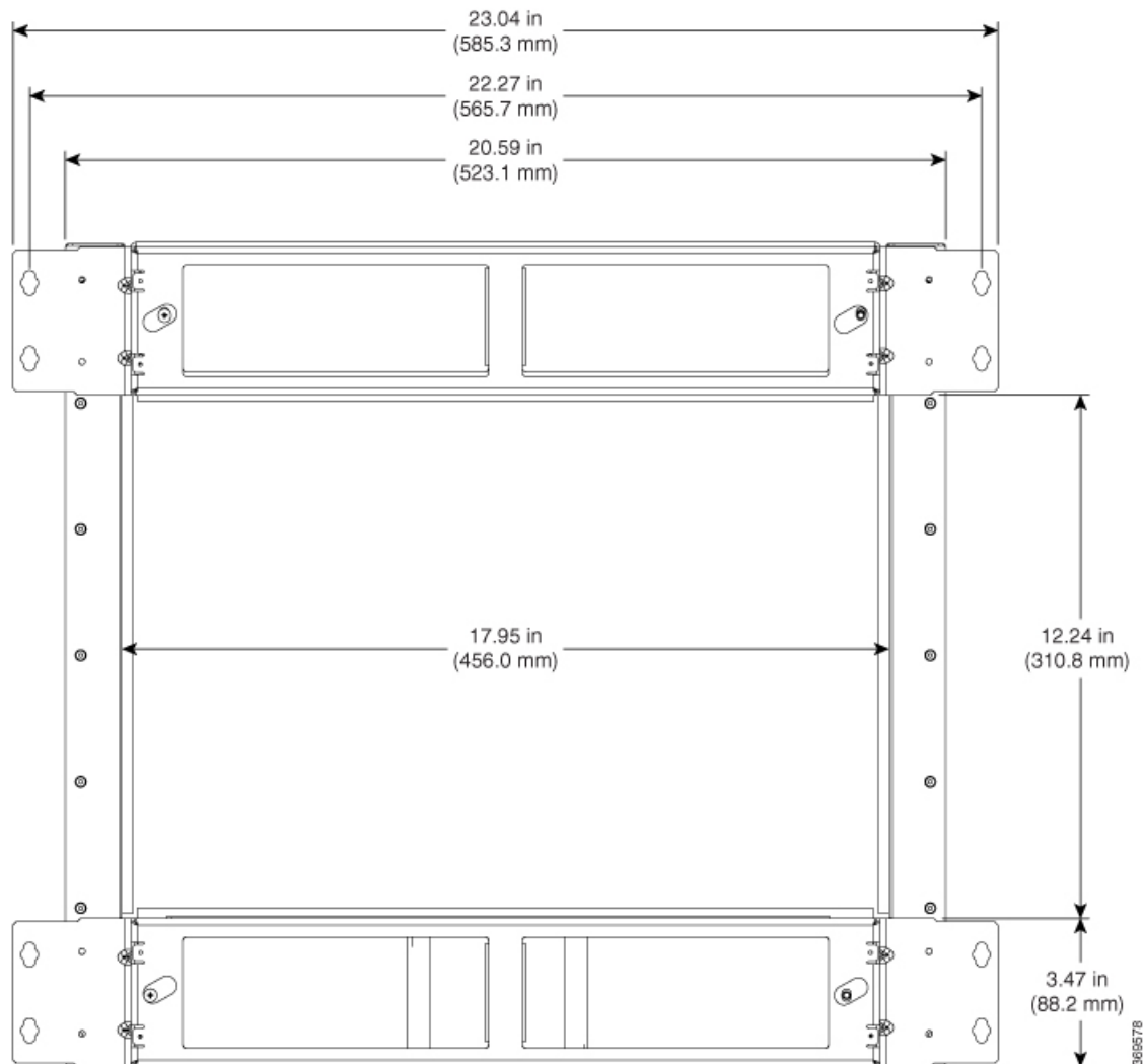
図 2: Cisco A907-F2B-AIR クリアランスの前面図
