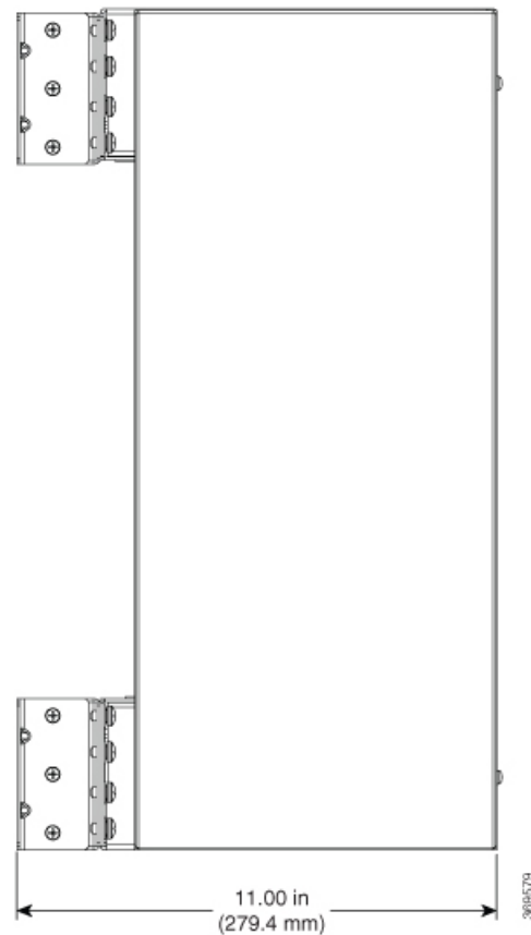
図 3: Cisco A907-F2B-AIR クリアランスの側面図
