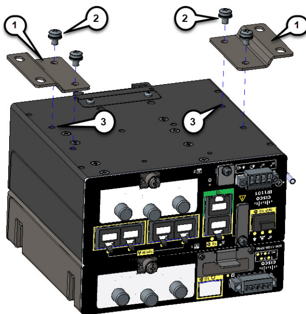
図 6: マウントブラケット
