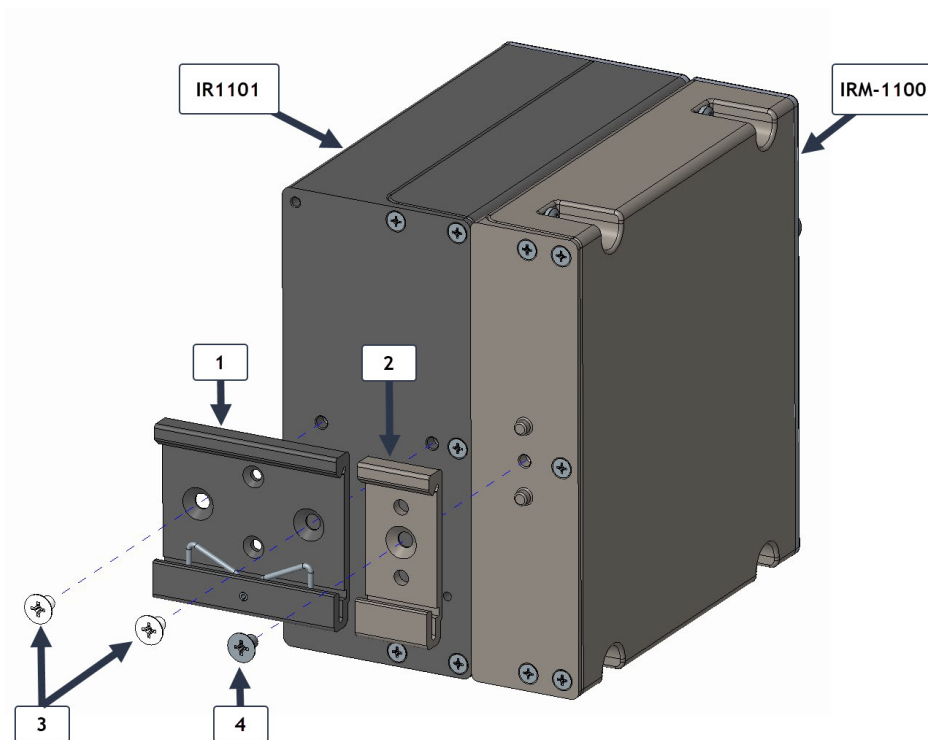
図 10: DIN レールブラケットの取り付け
