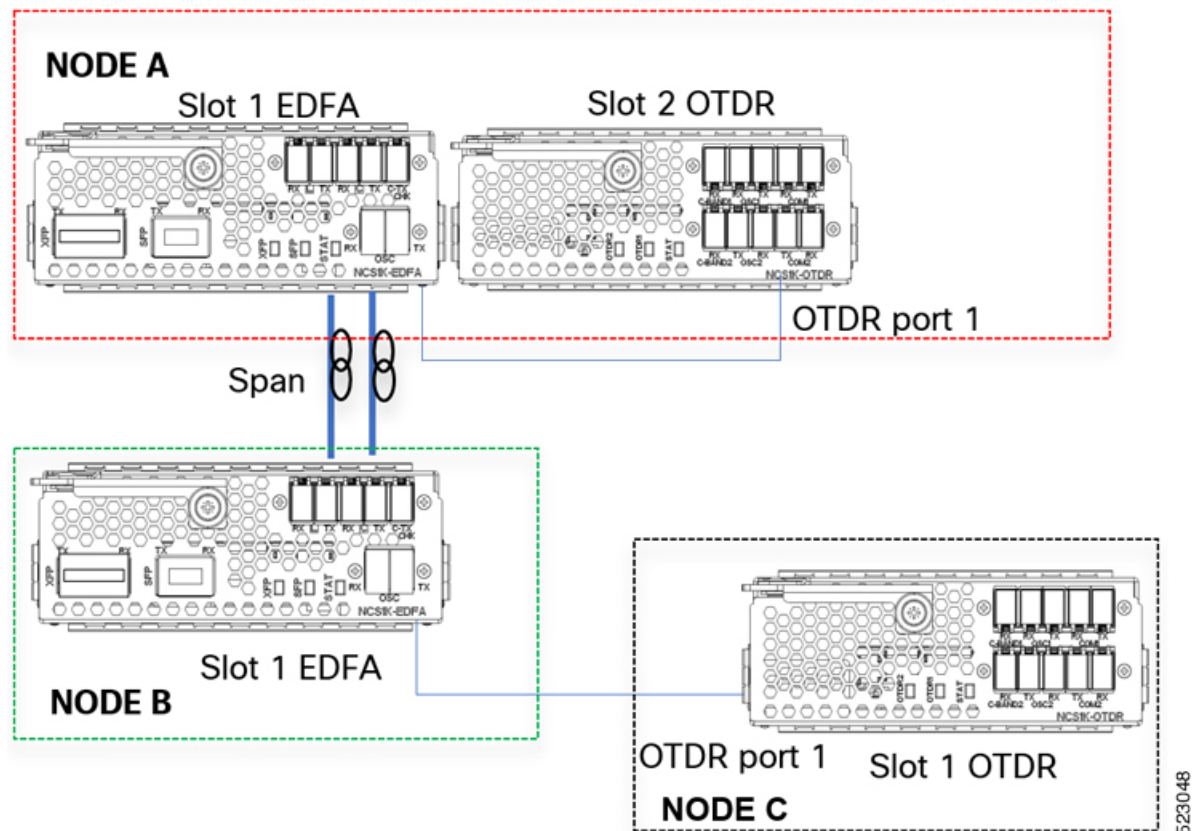
図 8: EDFA HW-module remote_node の設定
