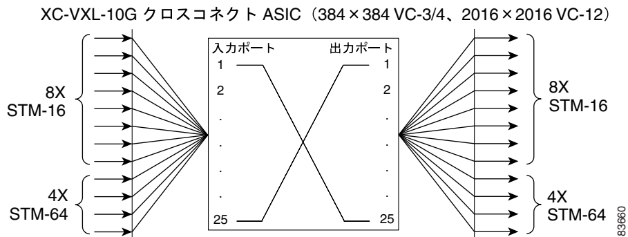
図 2-4 XC-VXL-10G のクロスコネクタマトリクス
