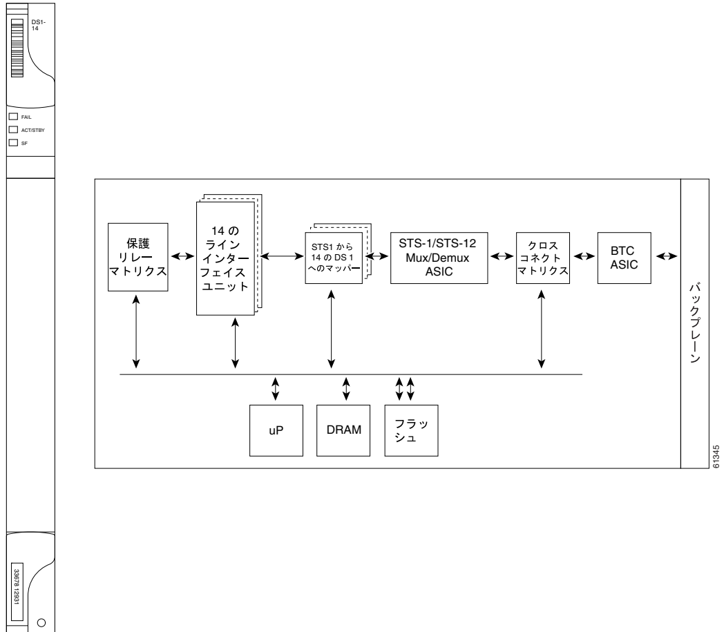
図 3-2 DS1-14 カードの前面プレートとブロック図
