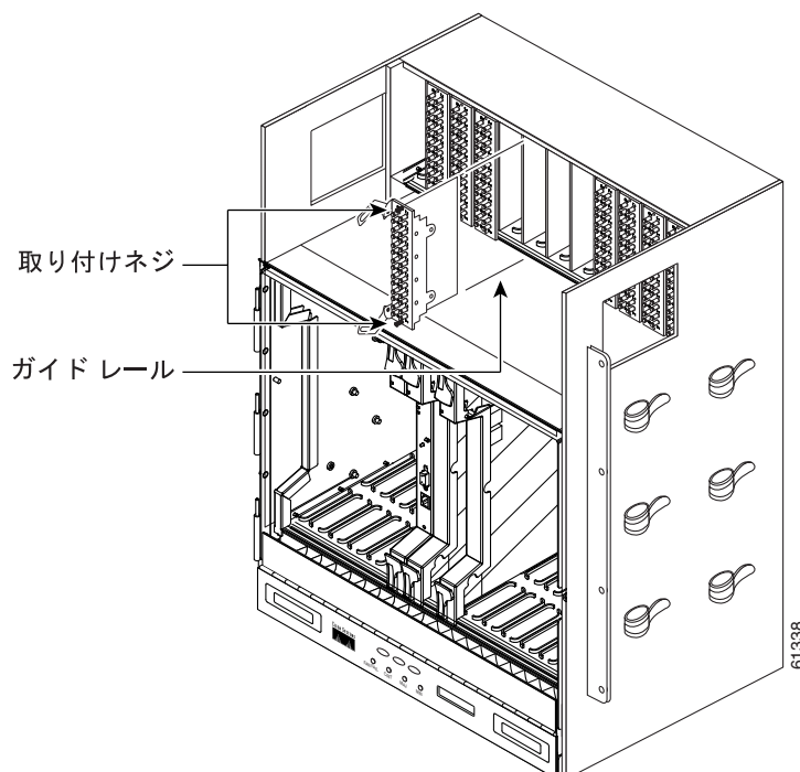
図 1-1 ONS 15454 SDH への FMEC の取り付け
