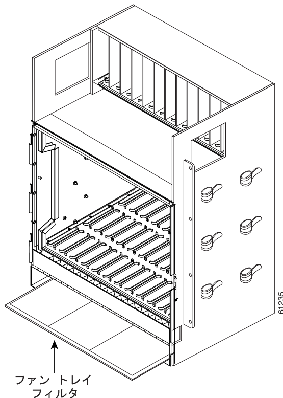
図 15-1 外部フィルタのブラケットに取り付けられている再使用可能なファントレイ エアー フィルタ (前面扉が取り外された状態)
