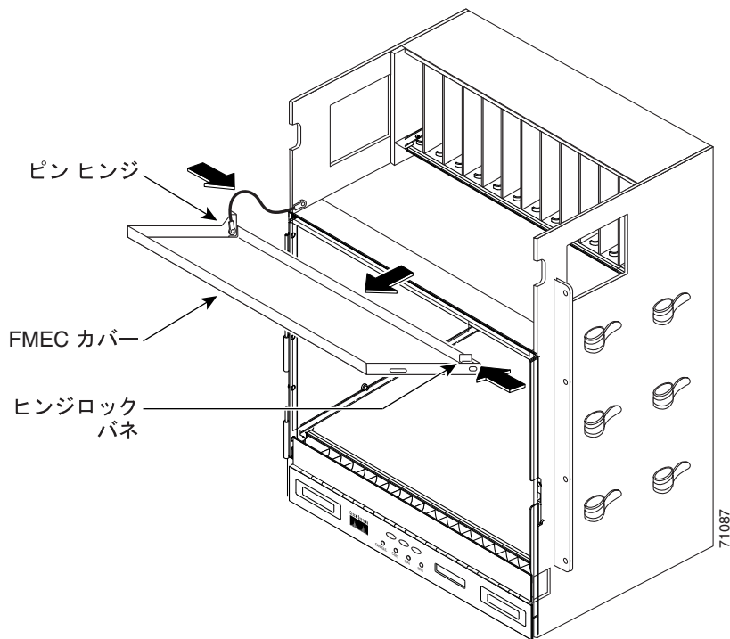
図 1-4 ONS 15454 SDH FMEC カバー
