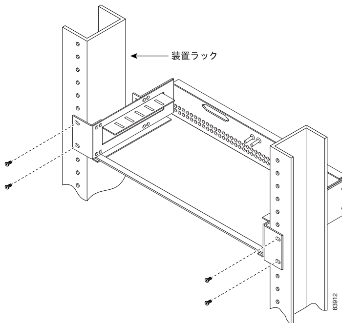
図 1-3 ラックへの E1-75/120 変換パネルの取り付け
