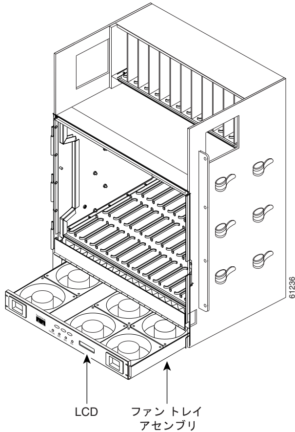
図 1-2 ファントレイ アセンブリの取り付け
