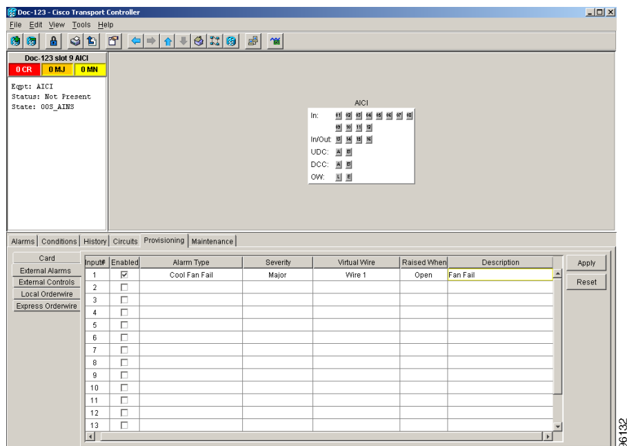
図 8-3 AIC-I カードでの外部アラームのプロビジョニング
