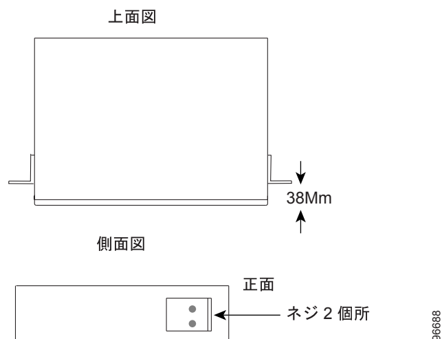
図 1 マウントブラケットの位置合わせ
