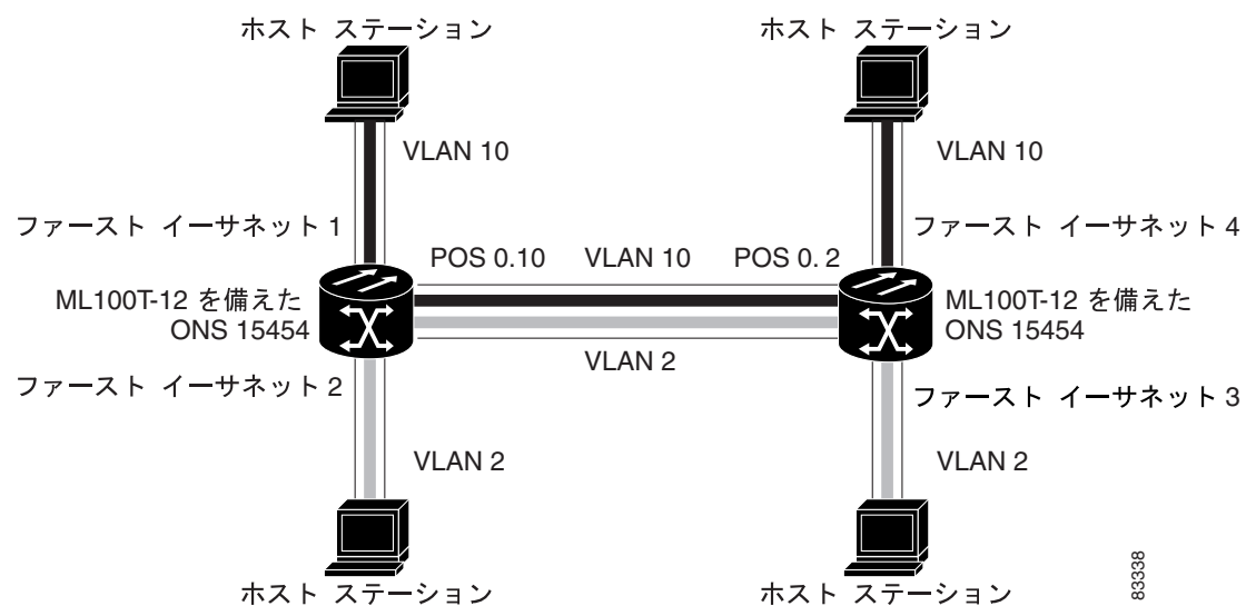
図 8-1 ネットワーク内の装置にまたがる VLAN
