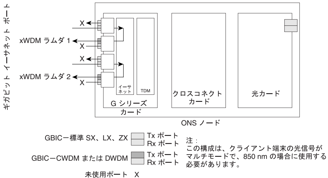
図 23-10 2 ポート単方向トランスポンダ
