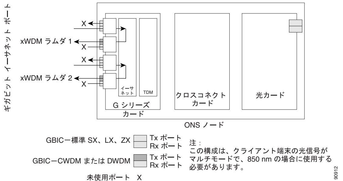
図 23-10 2 ポート単方向トランスポンダ
