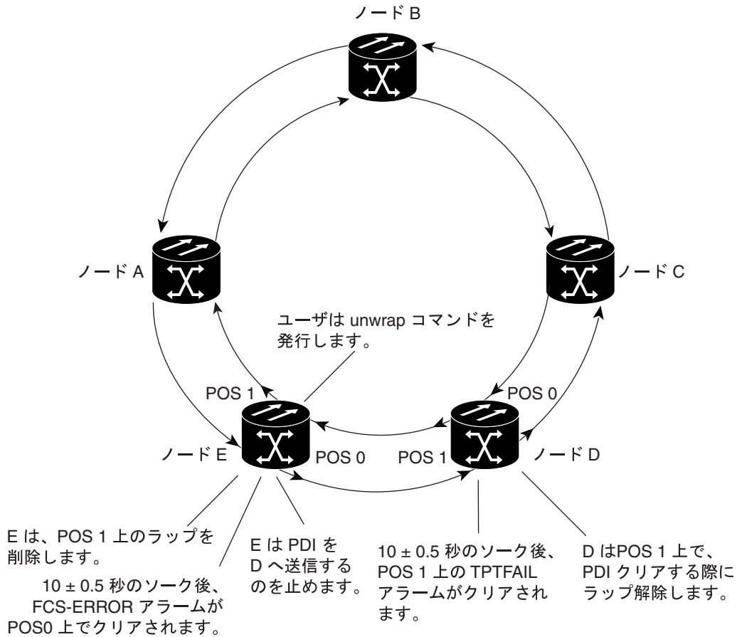
図 21-3 双方向の超過 CRC エラーでラップ解除された RPR
