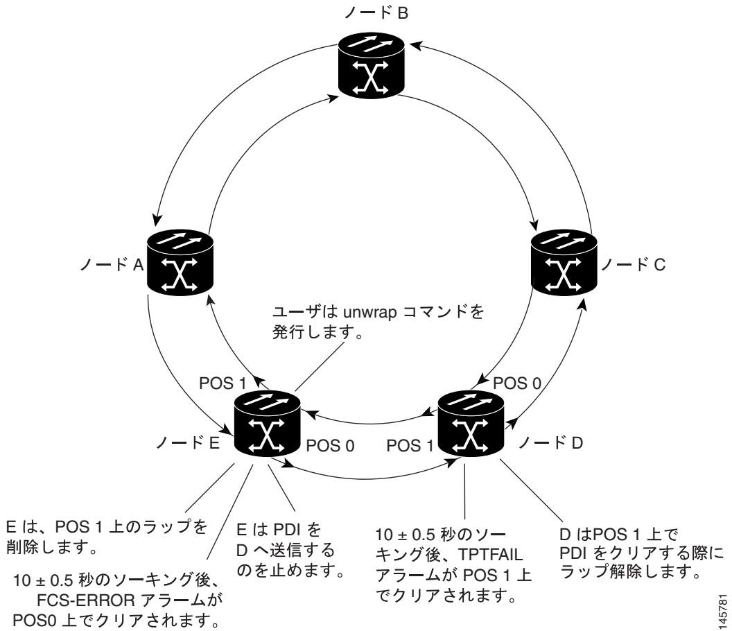
図 21-4 双方向の超過CRCエラーでラップされたRPR
