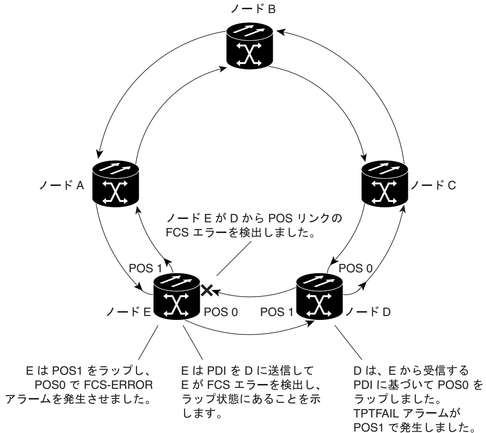
図 21-2 単一方向の超過 CRC エラーでラップされた RPR
