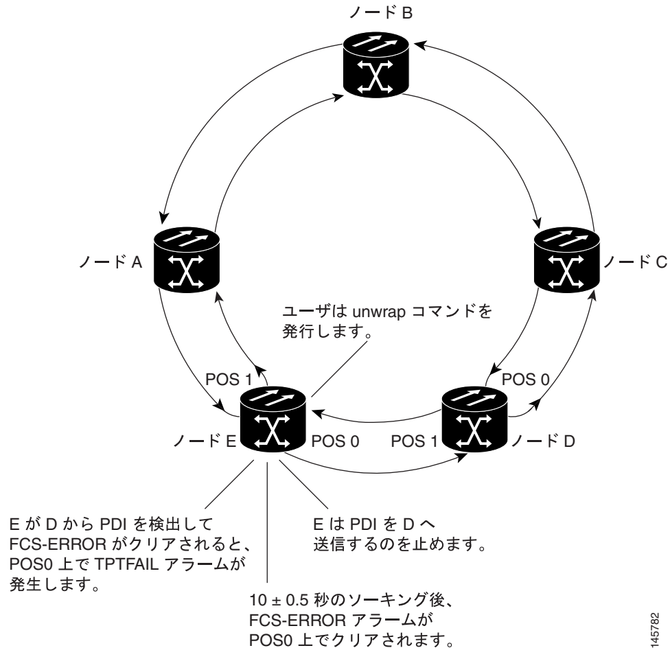
図 21-5 双方向の超過 CRC エラーでラップ解除された RPR の最初の段階
