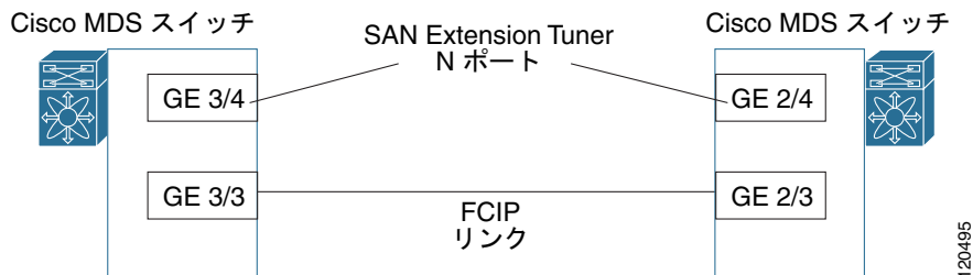
図 3-3 FCIP リンクに対応する N ポート調整の論理構成例
