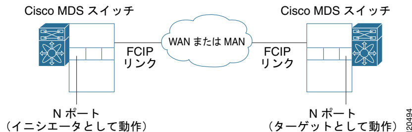
図 3-2 N ポート調整の物理構成例
