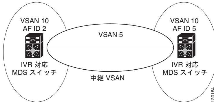
図 2-1 AFID を使用し、一意ではない VSAN ID を持つ IVR トポロジの例
