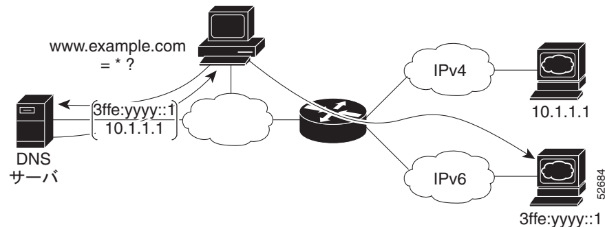
図 8-10 デュアル IPv4 および IPv6 プロトコル スタック アプリケーション
