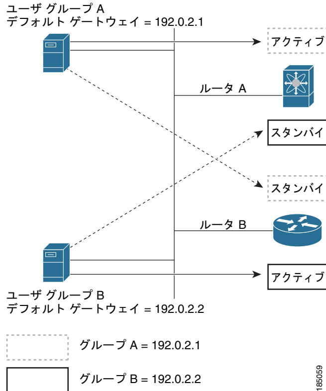
図 5-2 HSRP ロード シェアリング
