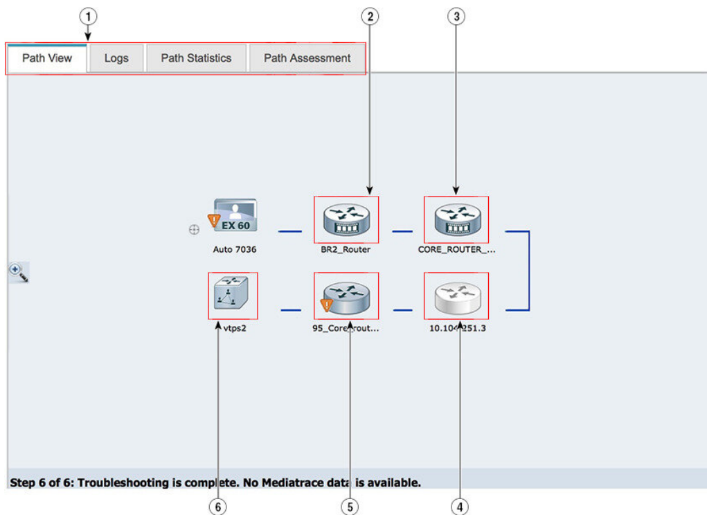
図 3: エンドポイント間のトラブルシューティング セッション
