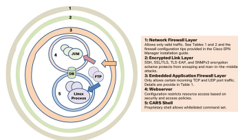
図 16: 複数レイヤで保護された境界アーキテクチャ：強化された外部シェルを備えた仮想アプライアンスシステム
