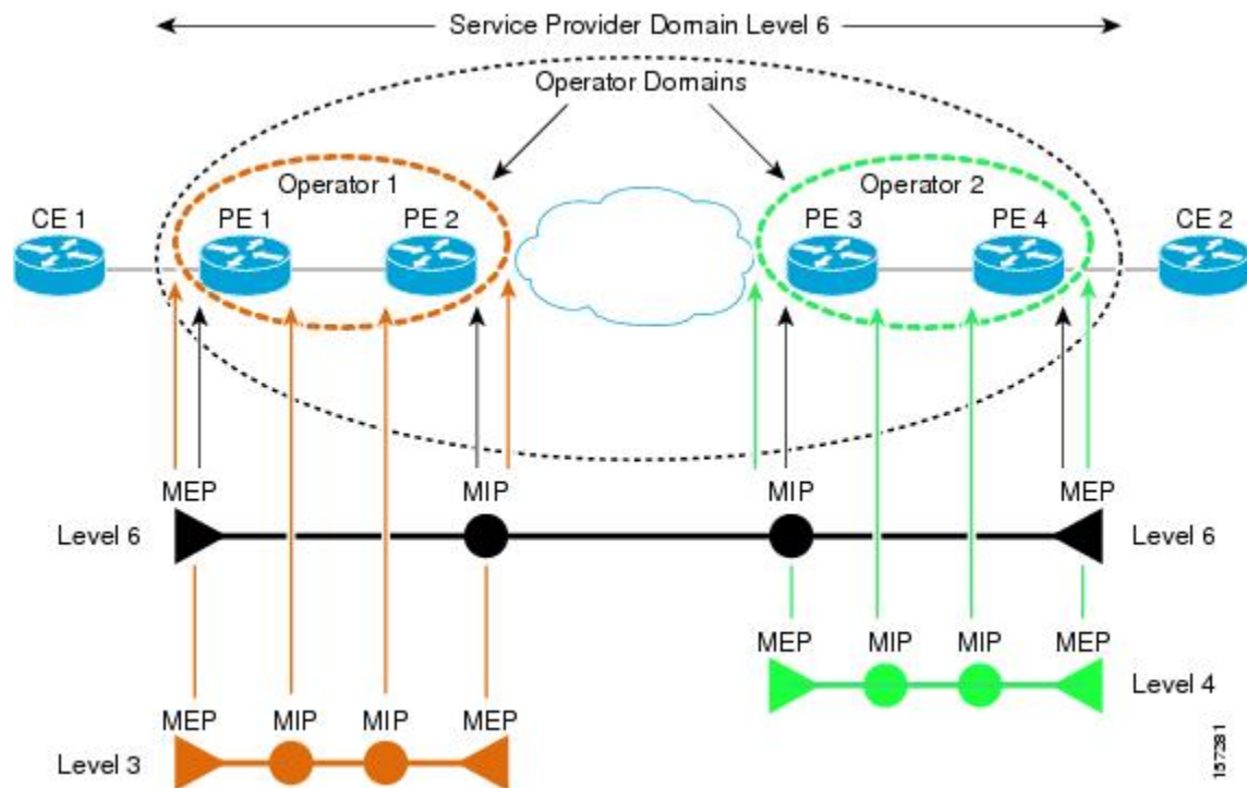
図 11: CFM メンテナンス ドメイン
