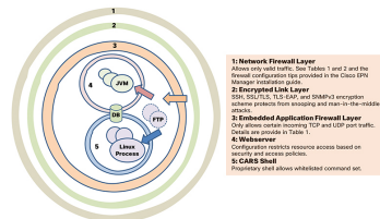
図 17: 複数レイヤで保護された境界アーキテクチャ: 強化された外部シェルを備えた仮想アプライアンスシステム
