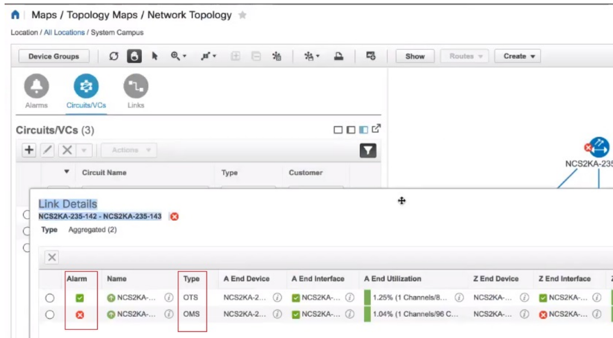
図 4: アラームを使用した [リンクの詳細 (Link Details)]
