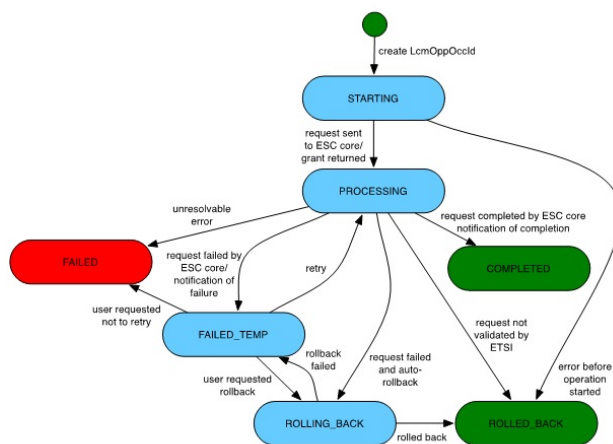
図 1: VNF ライフサイクル管理の遷移状態
