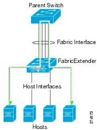
Figure 1: 転送モデル
