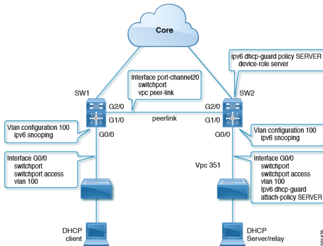
Figure 14: 孤立ポート上のクライアントおよび DHCP リレーによる FHS 設定
