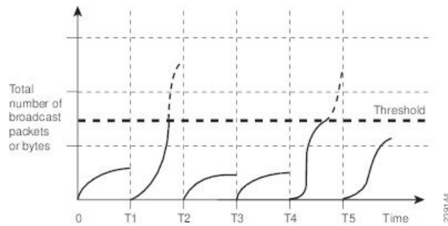
Figure 18: ブロードキャストの抑制
