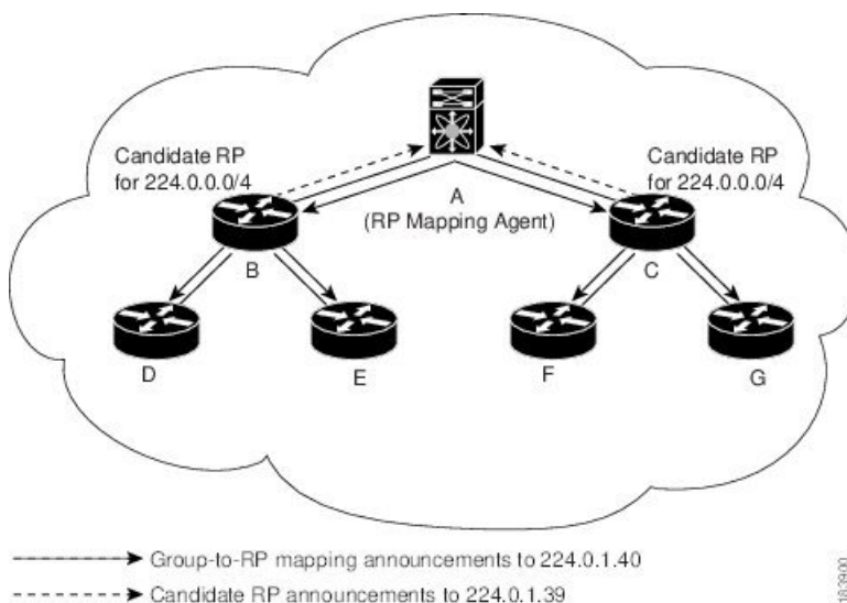
図 13: Auto-RP のメカニズム
