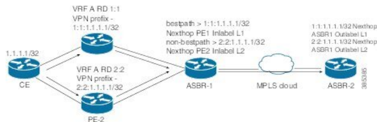
図 8: 個別のルート識別子を使用して構成された各 PE での仮想ルーティングおよび転送 (VRF)
