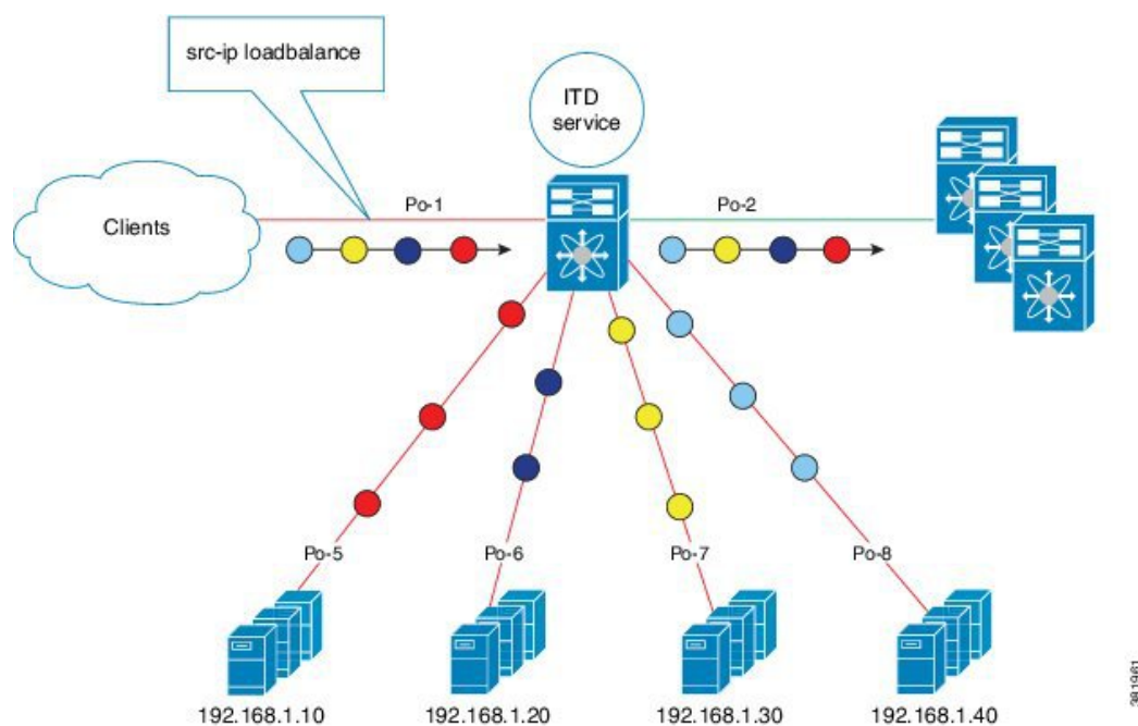
図 14: ワンアーム展開モード
