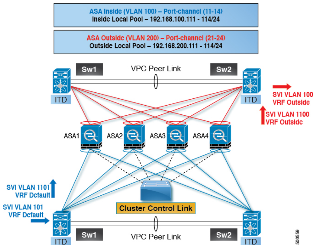
図 25: vPC を使用したデュアルスイッチ サンドイッチを備えた ASA クラス
