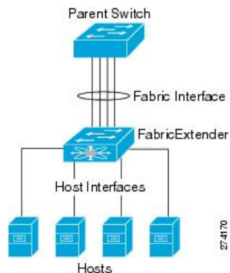
Figure 2: ポート チャンネル ファブリック インターフェイス 接続
