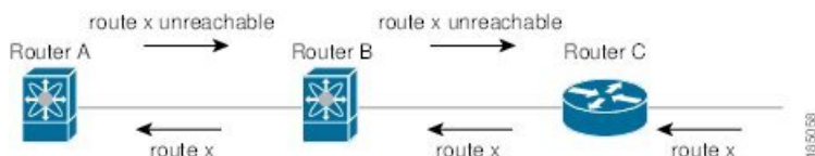
図 33: スプリット ホライズン ポイズン リバーズを指定した RIP
