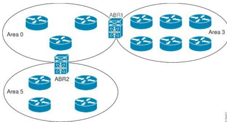
図 23: OSPFv3 エリア
