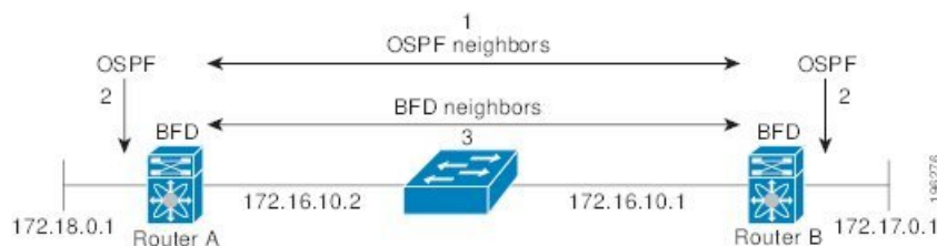
図 6: BFD ネイバー関係の確立
