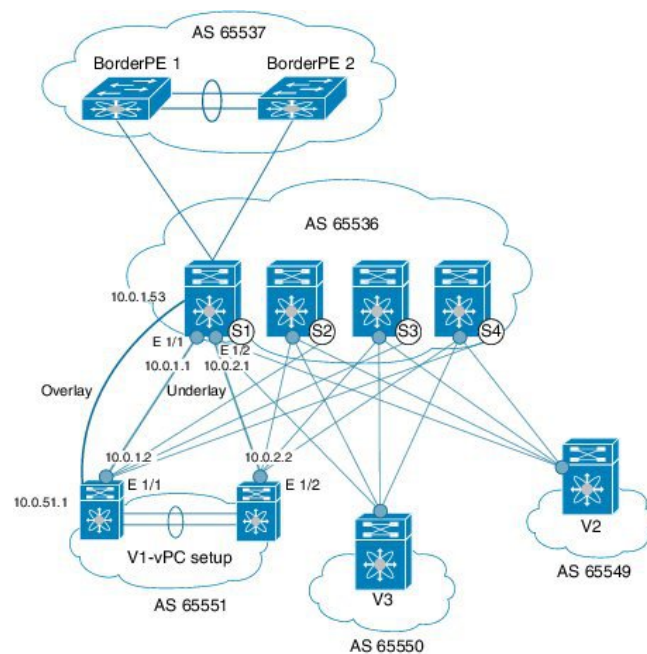
図 5: アンダーレイとしての eBGP
