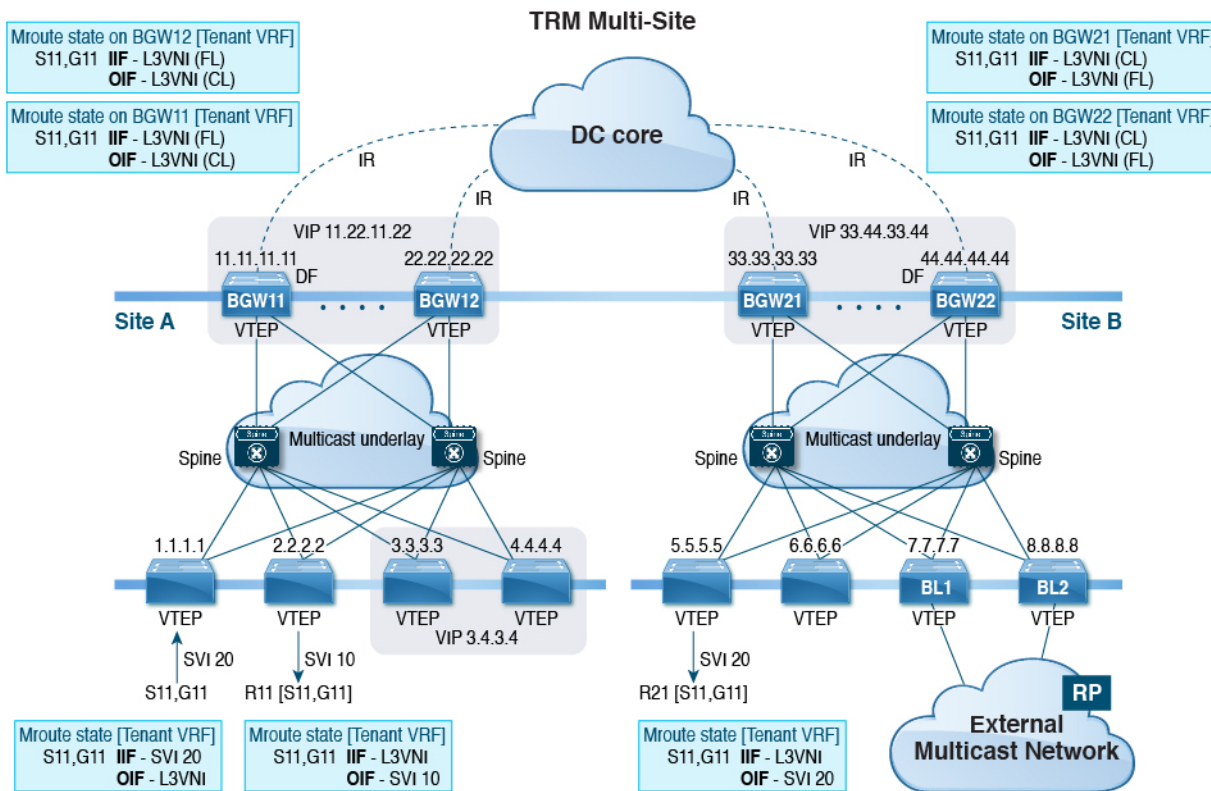
図 1: マルチサイトトポロジの TRM、BL 外部マルチキャスト接続
