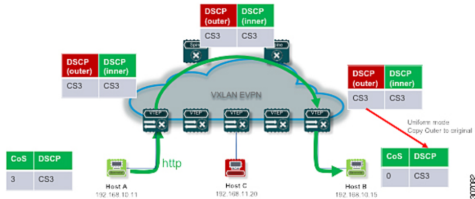
図 39: ユニフォーム モードの外部 DSCP 値がレイヤ 3 パケットのカプセル化解除されたパケット DSCP 値にコピーされる
