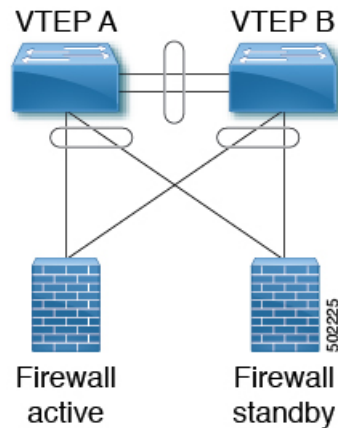
図 51: 静的ルーティングを使用するデュアル接続ファイアウォール
