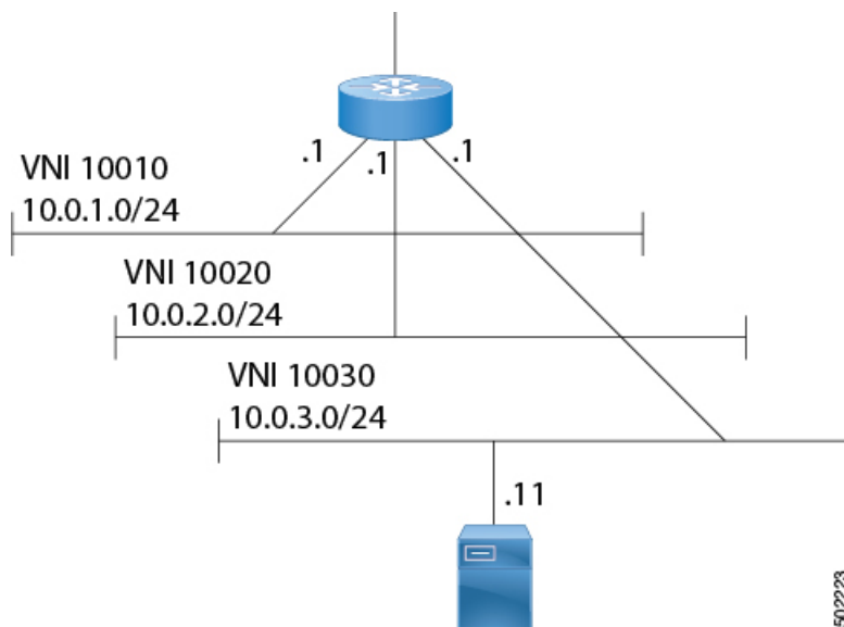
図 55: レイヤ 2 VXLAN ファブリックを使用したデフォルト ゲートウェイとしてのファイアウォール
