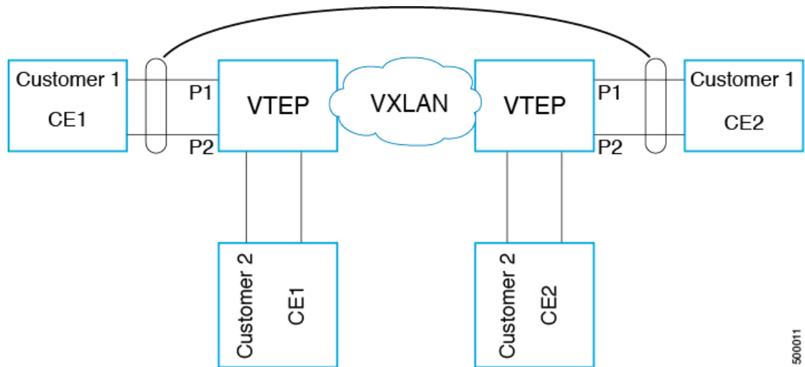
図 31: VXLAN P2P トンネルを通じた LACP トンネリング
