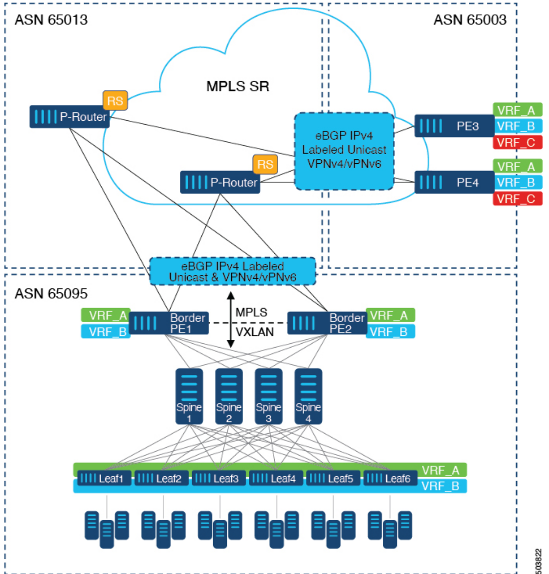
図 42: コアネットワーク内の複数の管理ドメイン
