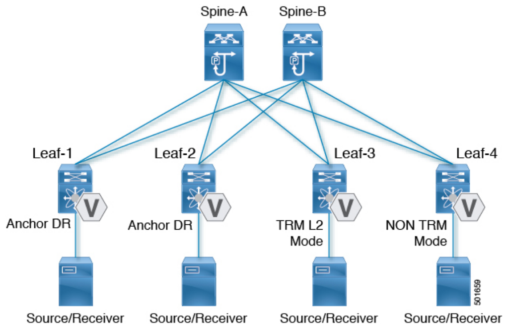
図 30: TRM レイヤ 2/レイヤ 3 混合モード
