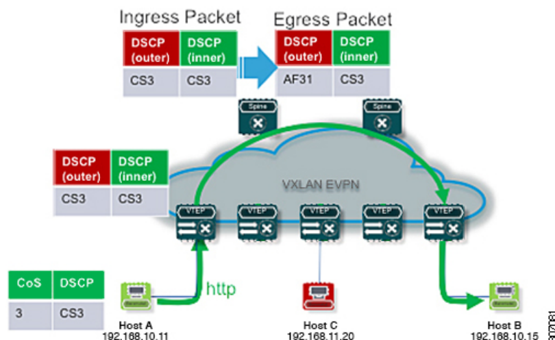
図 38: VXLAN トンネル内部のマーキング
