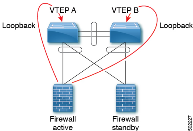
図 53: eBGP を使用したデュアル接続ファイアウォール
