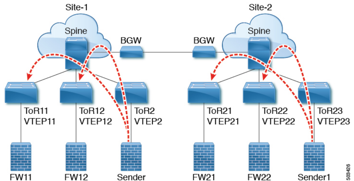
図 58: マルチサイト トポロジでの VNF の比例マルチパス
