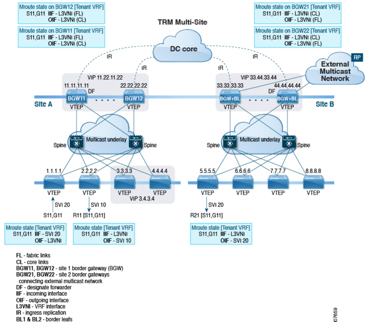
図 28: マルチサイト トポロジ、BGW 外部マルチキャスト接続を備えた TRM
