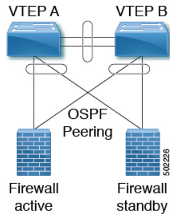
図 54: OSPF を使用したデュアル接続ファイアウォール
