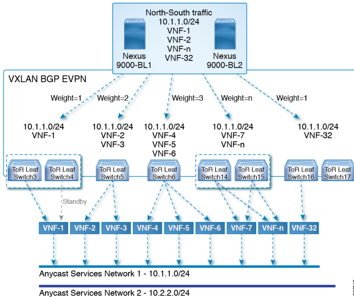
図 56: サンプル トポロジ (North-South トラフィック)
