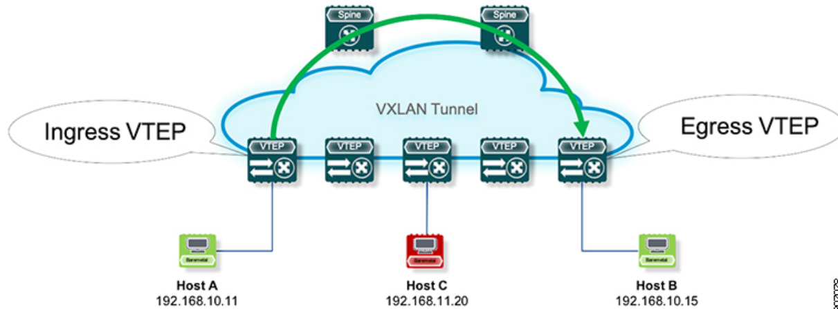
図 35: VXLAN ネットワーク
