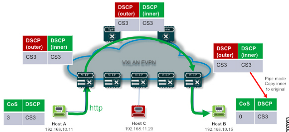
図 40: パイプモードの内部 DSCP 値がレイヤ 3 パケットのカプセル化解除されたパケット DSCP 値にコピーされる
