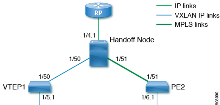
図 47: EVPN (TRM) と MVPN のシームレスな統合のサンプルトポロジ
