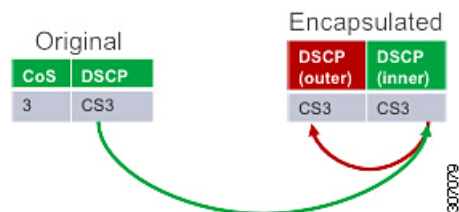
図 36: レイヤ 3 パケットから VXLAN 外部ヘッダーへの優先順位のコピー
