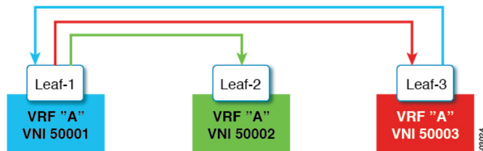
図 11: 非対称 VNI
