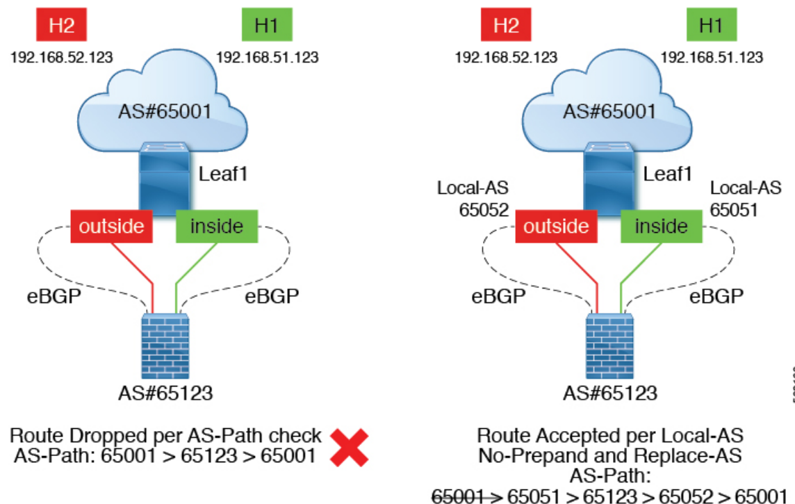
図 52: eBGP AS-Path チェック
