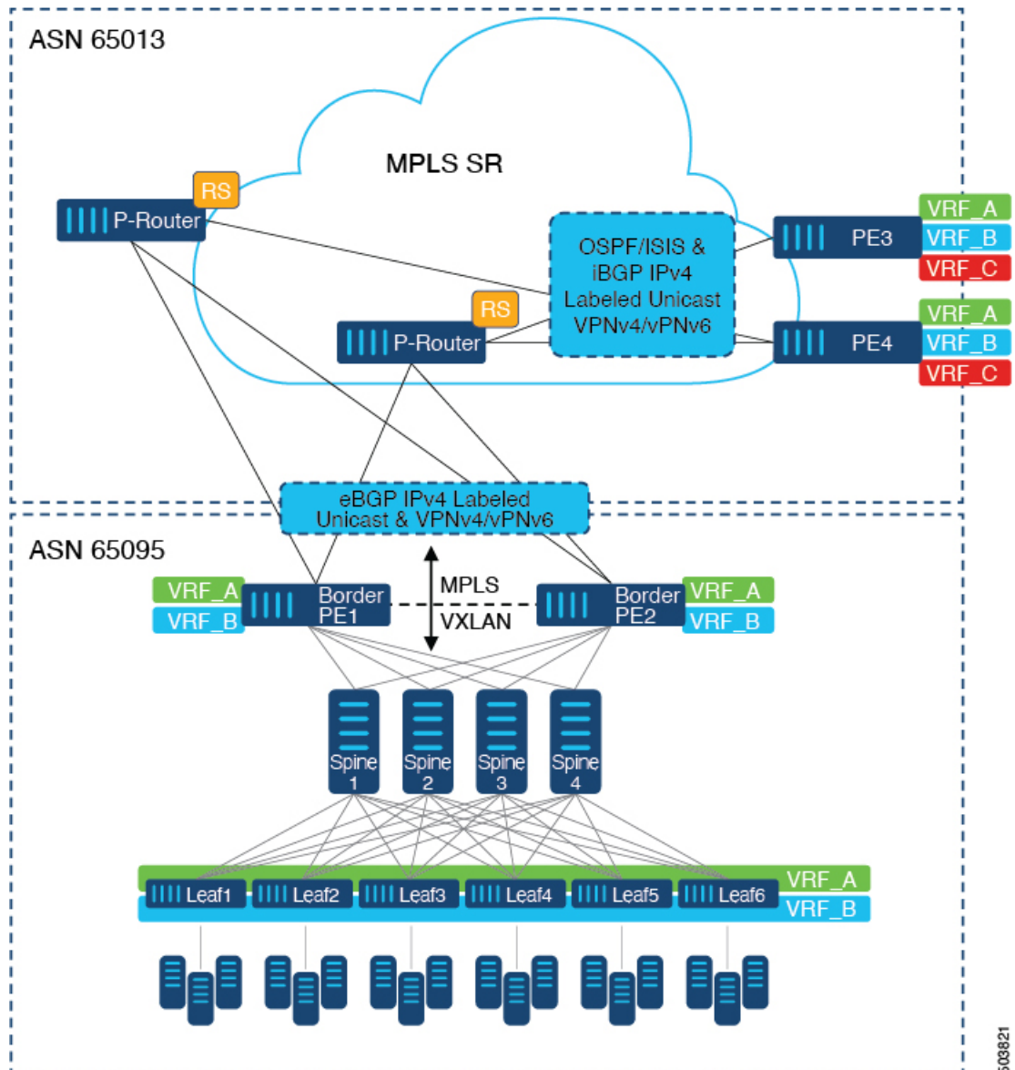
図 41: DCからコアネットワークドメインへの分離を使用したトポロジ
